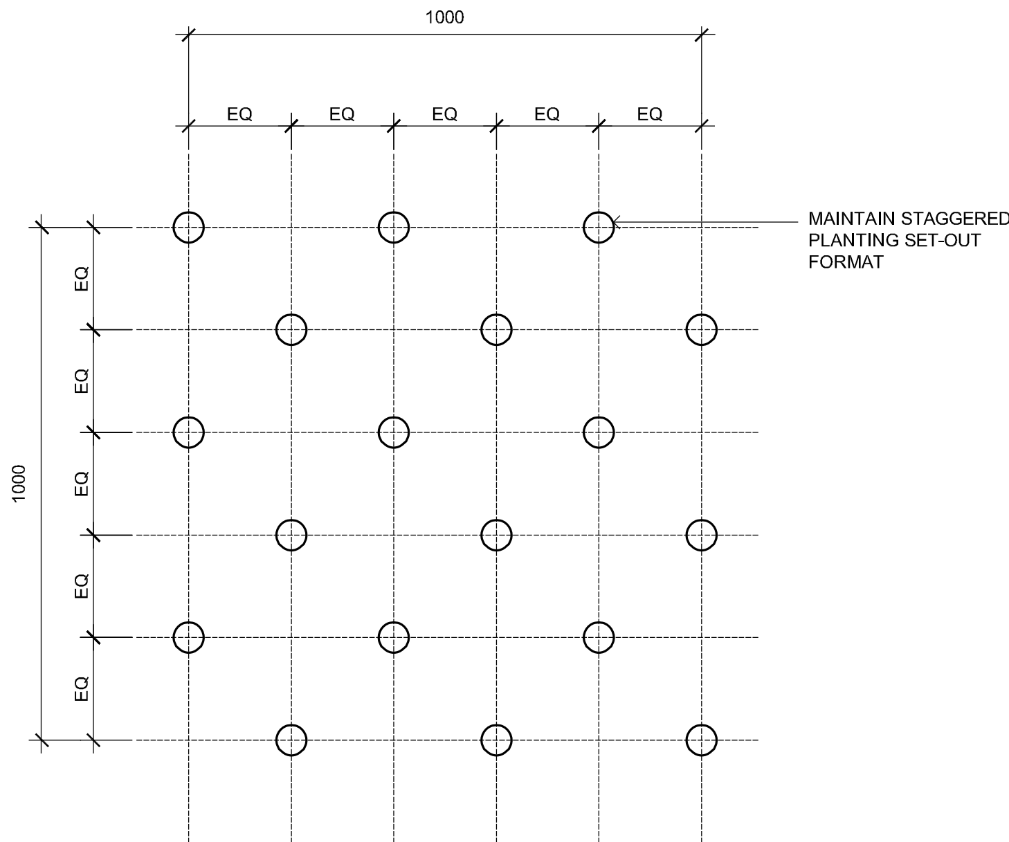
08 BIO-RETENTION MATRIX PLANTING SETOUT 501 N.T.S.
