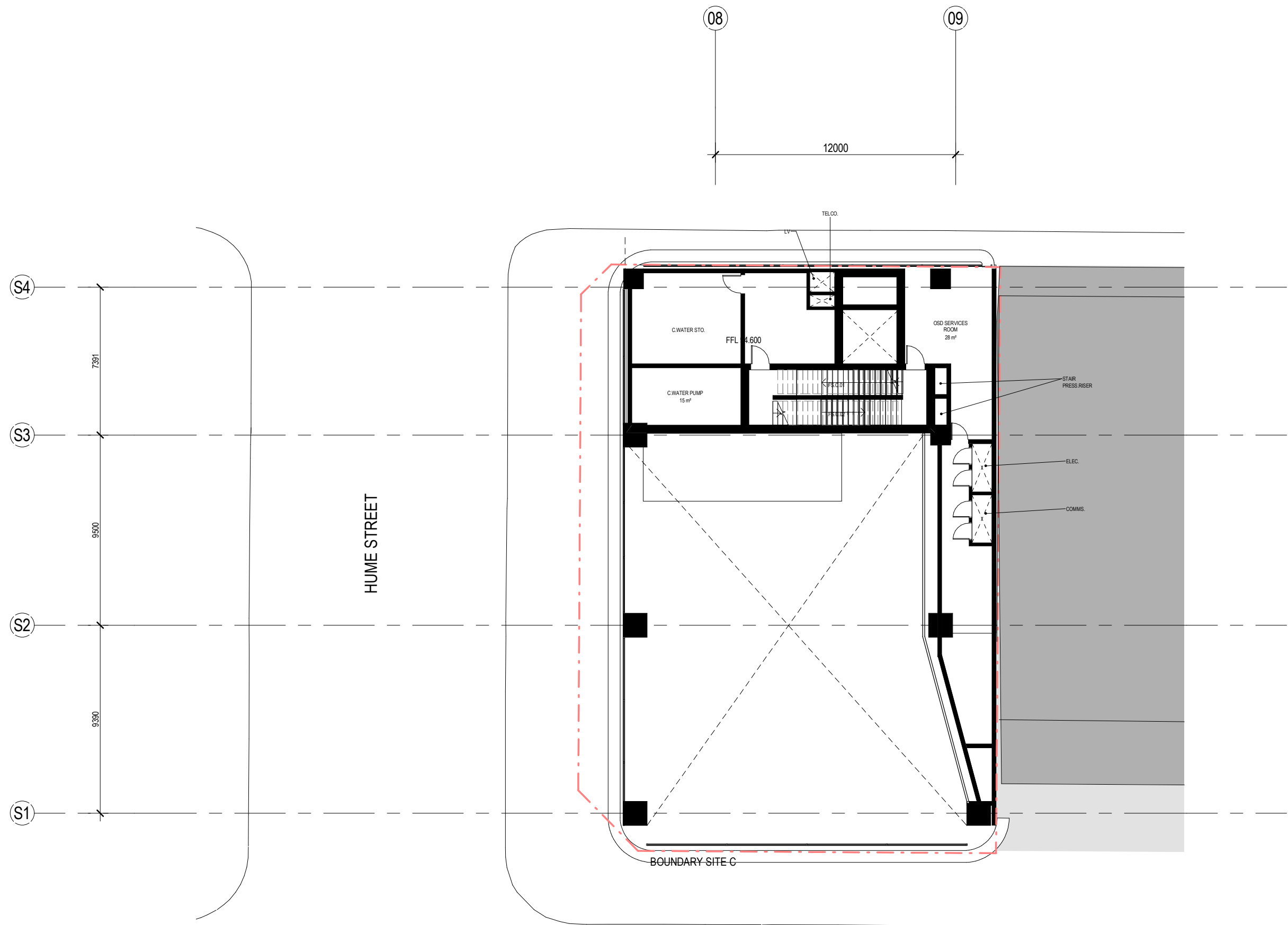
1 LEVEL 01 - SITE A / LEVEL 01 - SITE C 1:200
