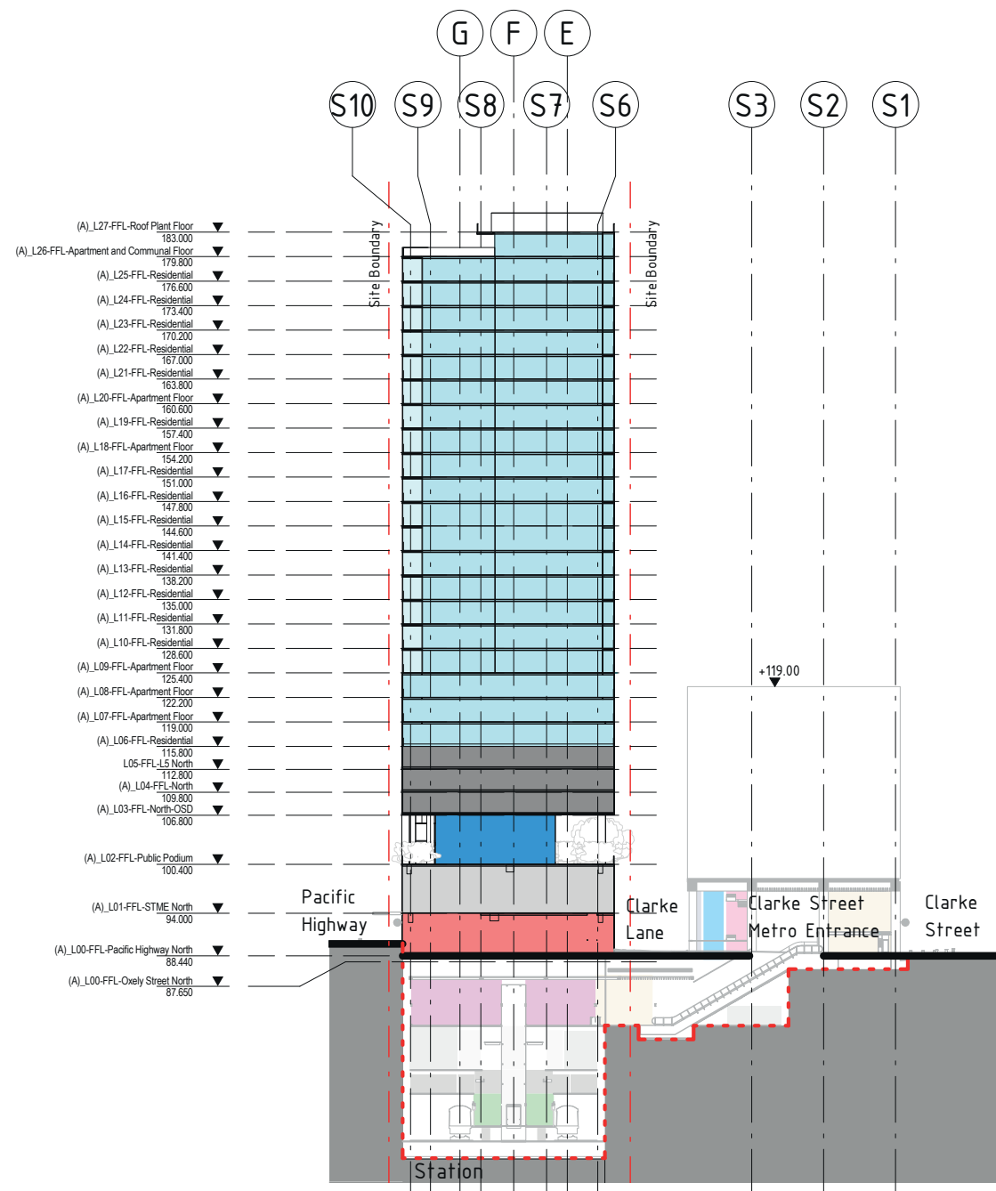
1 Cross Section Site A 1 : 1000
