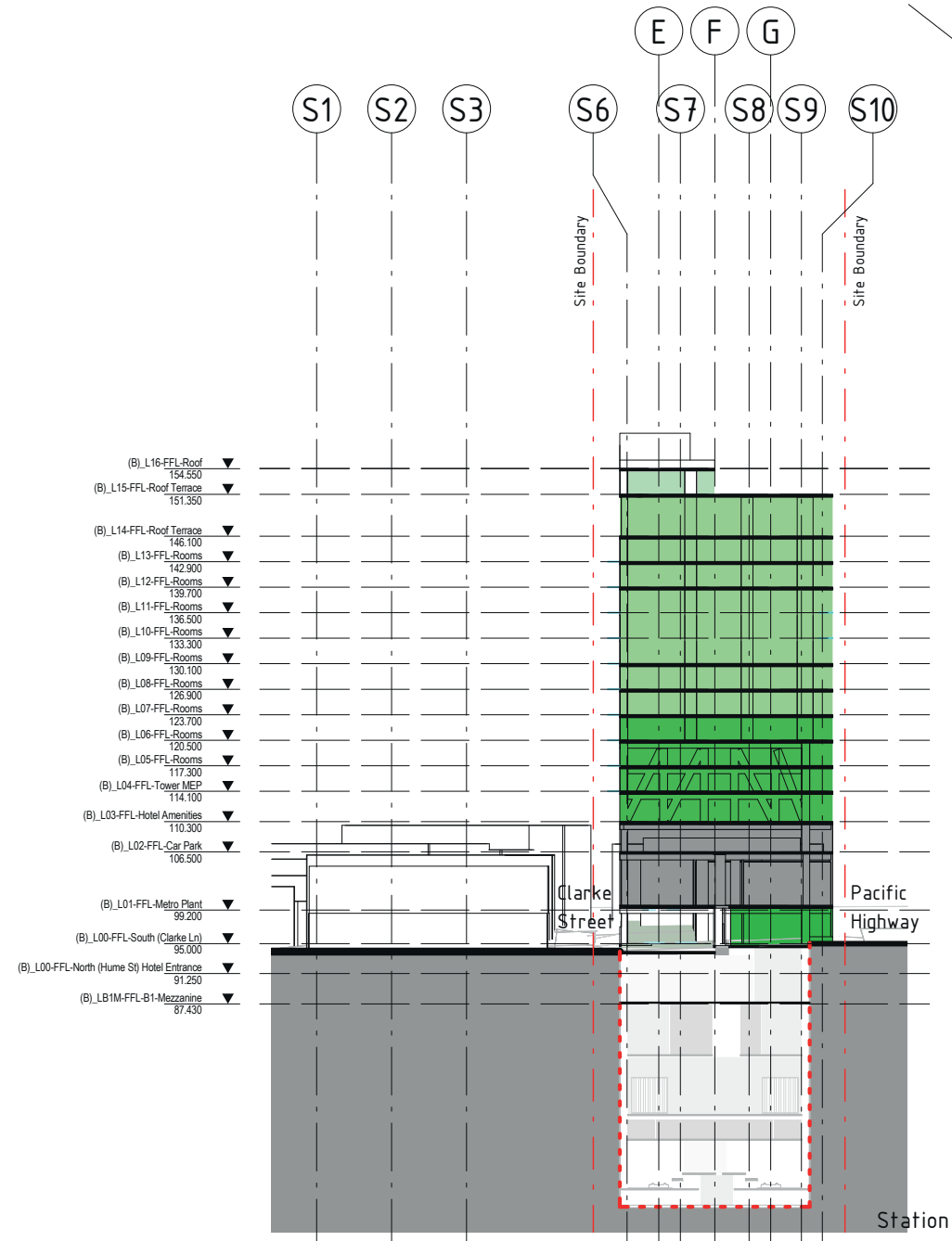
2 Cross Section Site B 1 : 1000
