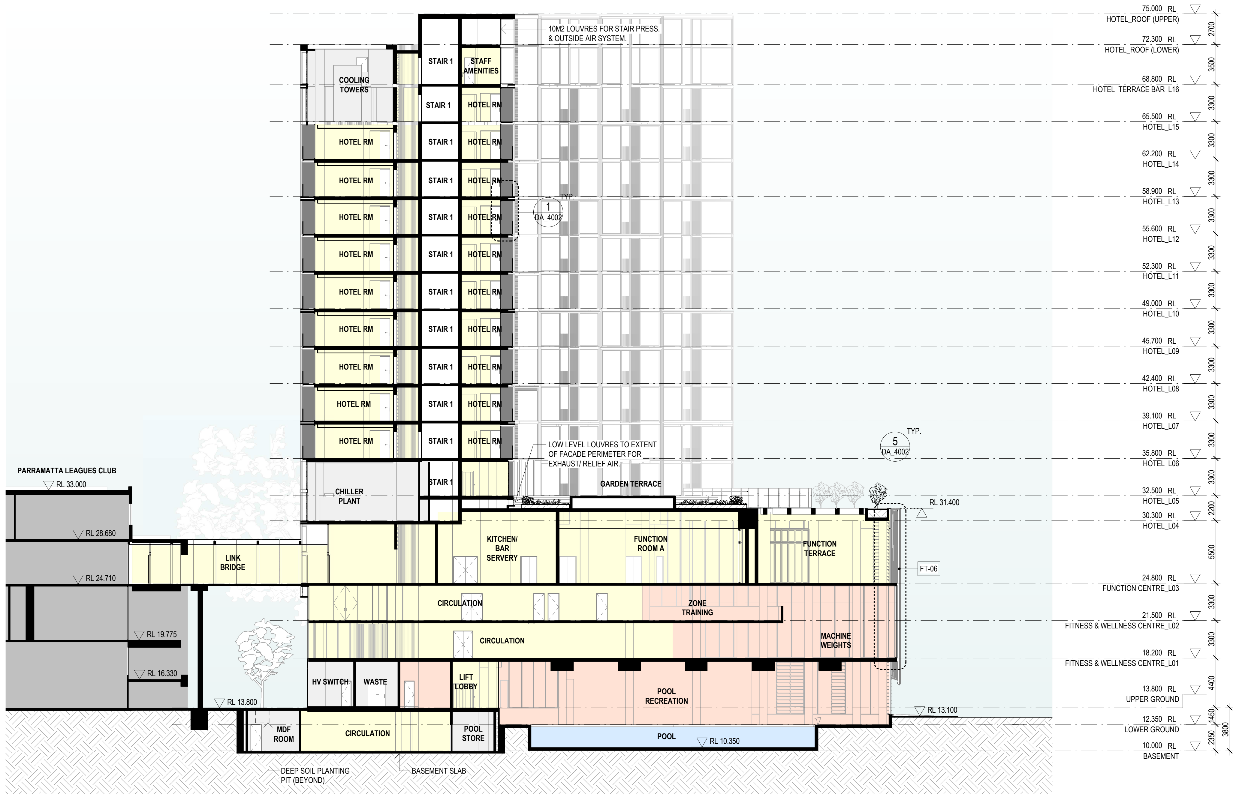
1 GA SECTION 1 DA_1100 1:200
