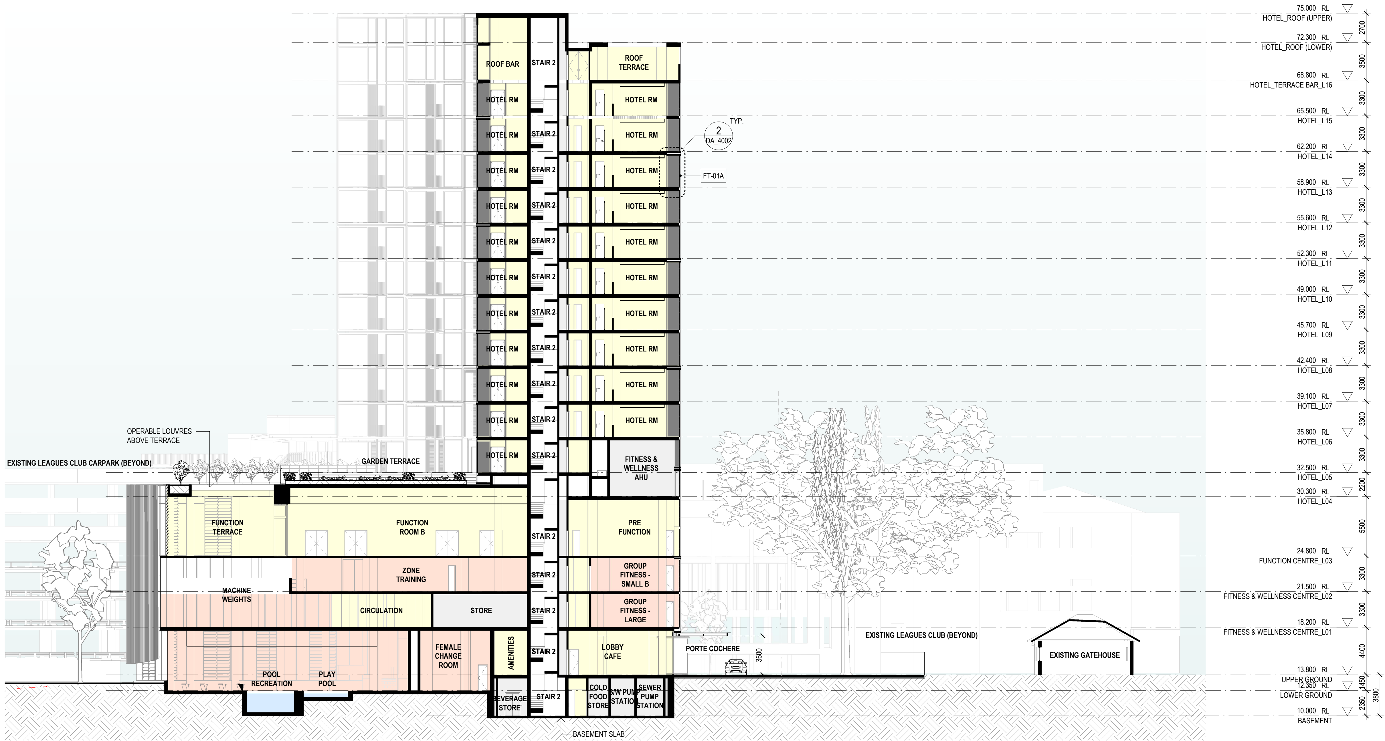
1 GA SECTION 2 DA_1100 1:200
