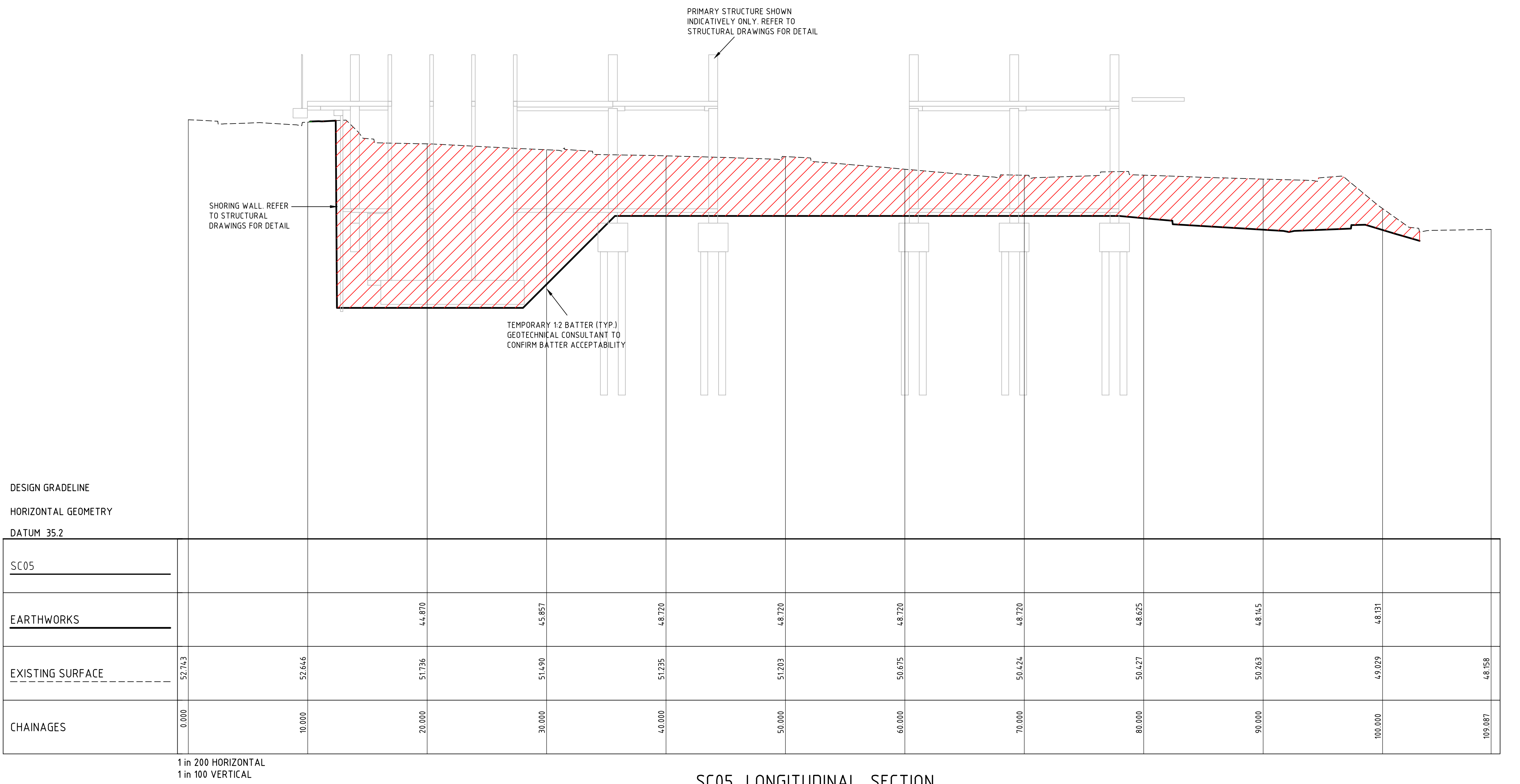
SC05 LONGITUDINAL SECTION
