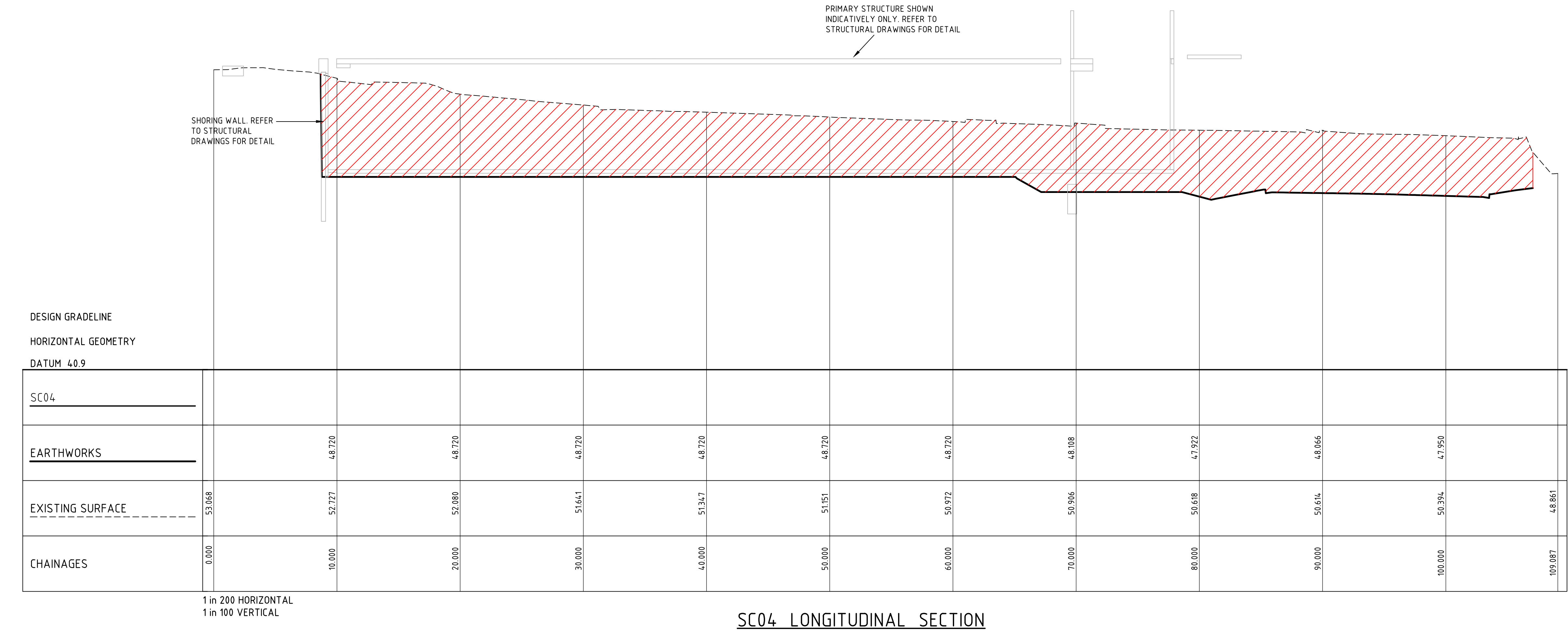
SC04 LONGITUDINAL SECTION
