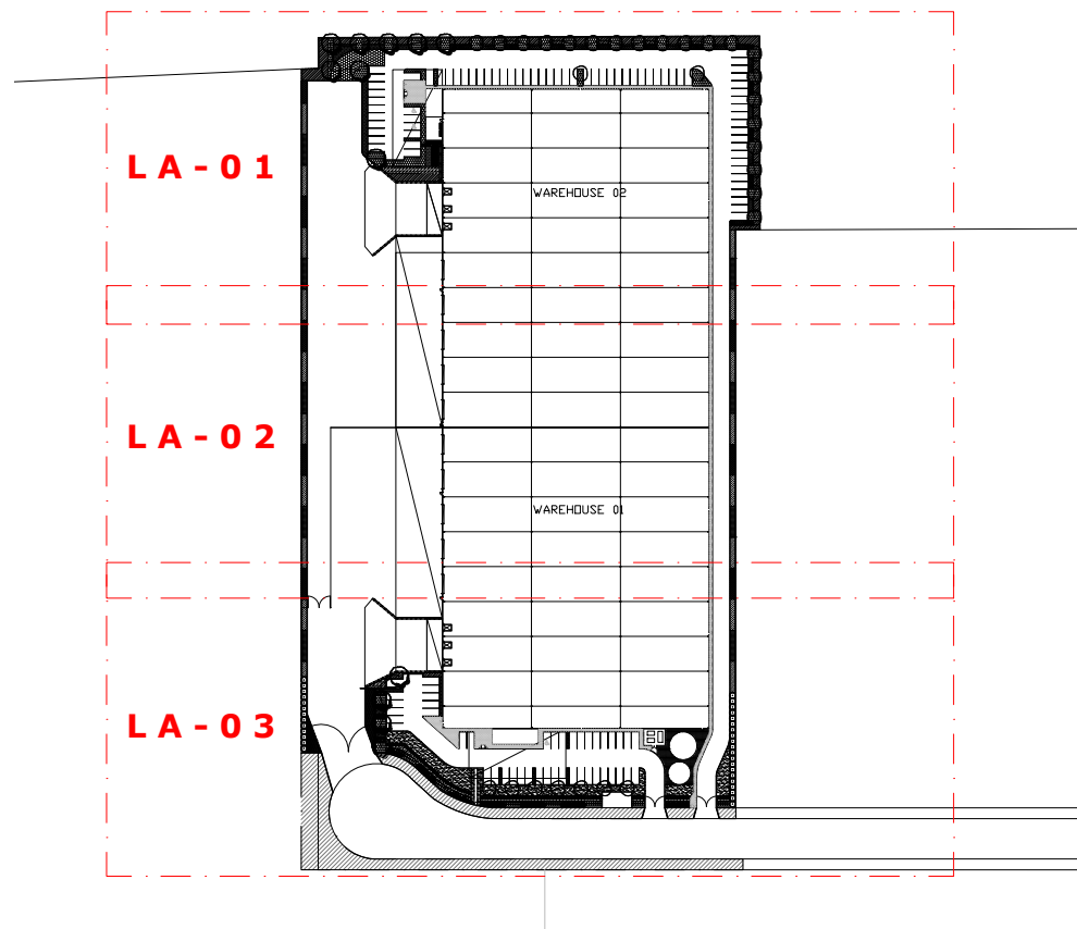
SITE LAYOUT SCALE - N.T.S.
