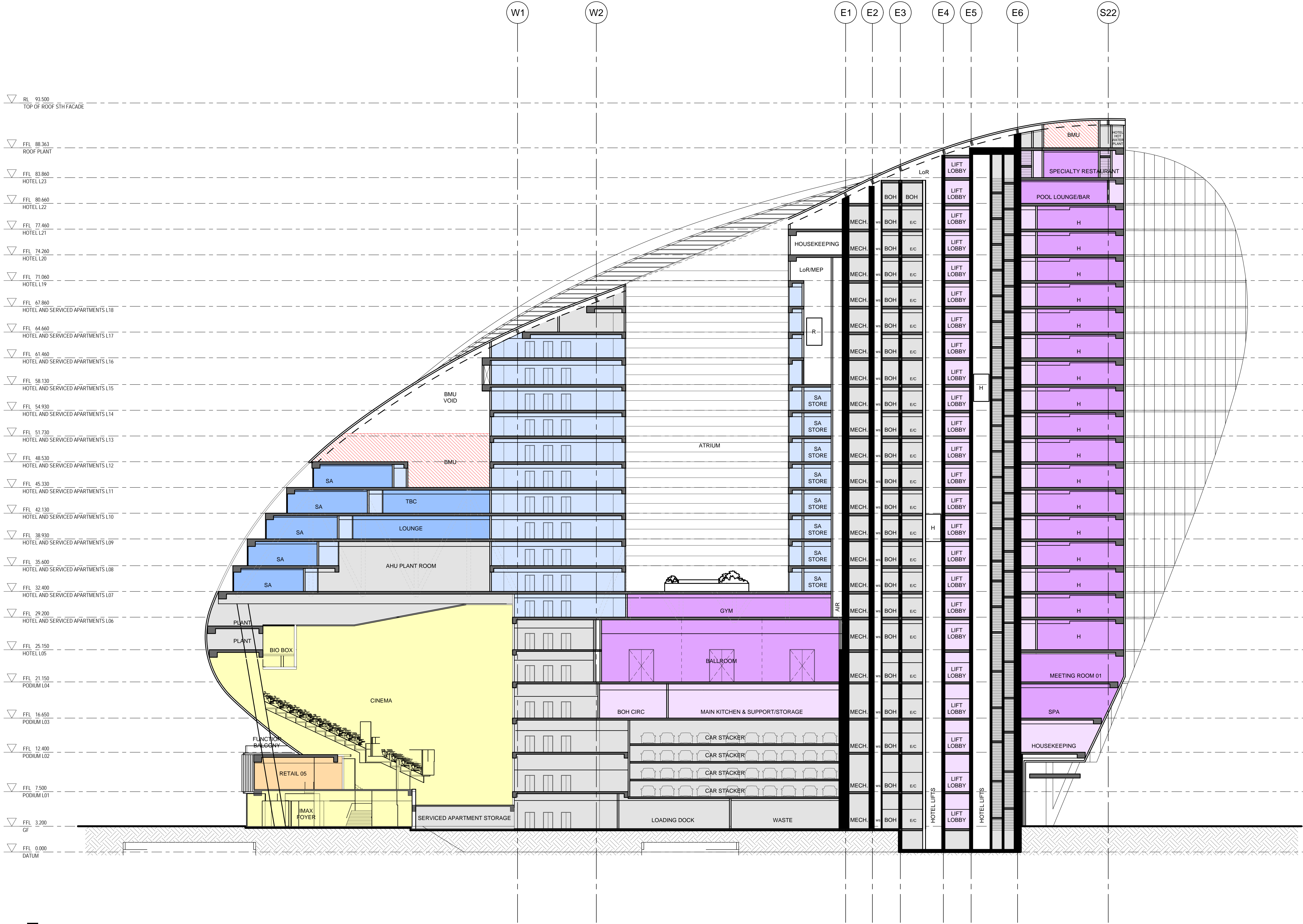
E SECTION 1:200
