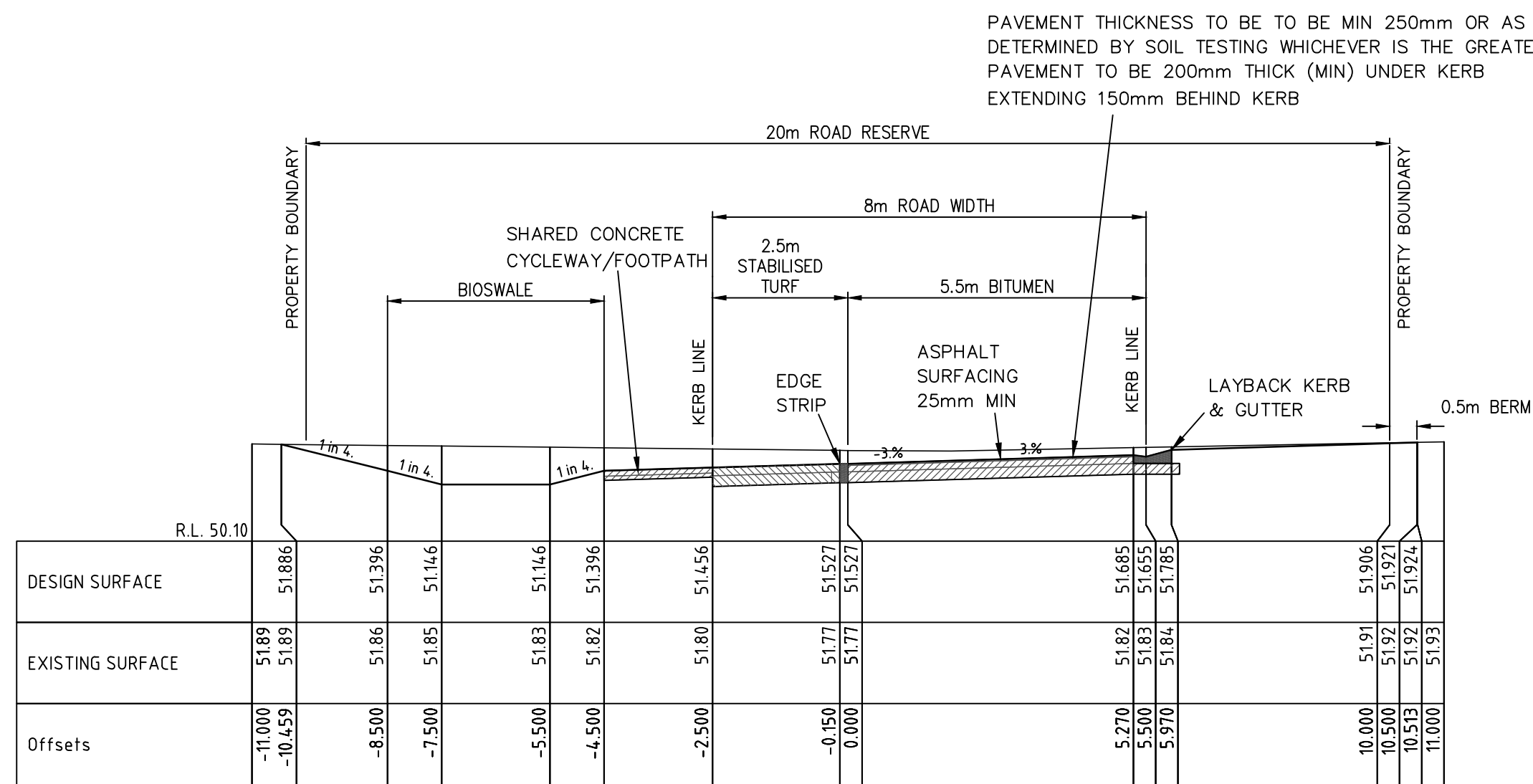
Ch 150. ROAD No. 16 Scale: 1 in100
