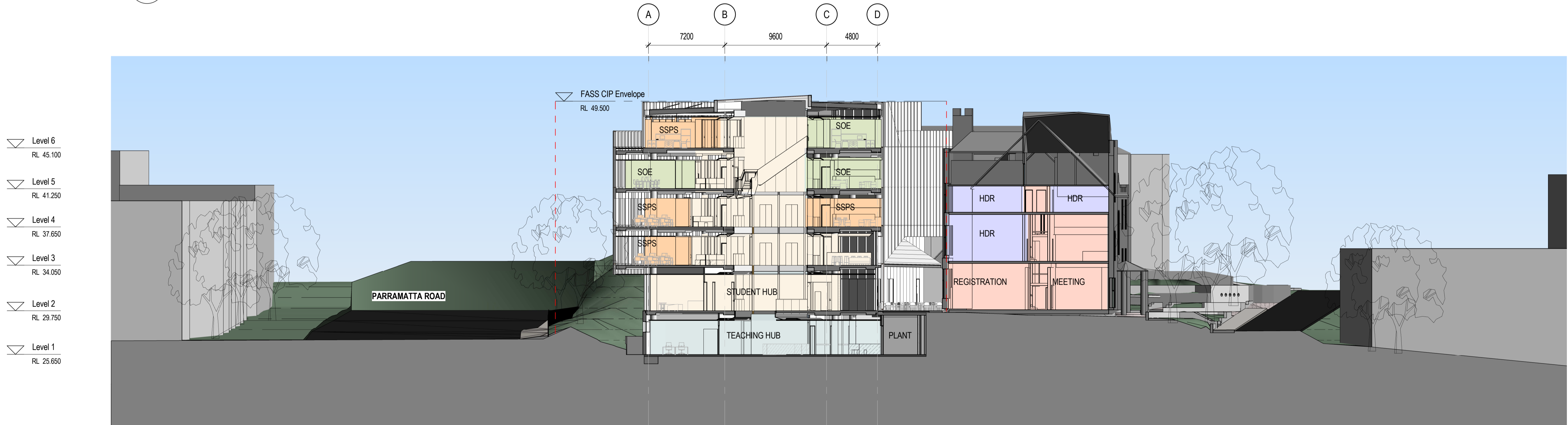
B Section B DA1010 Scale: 1 : 200
