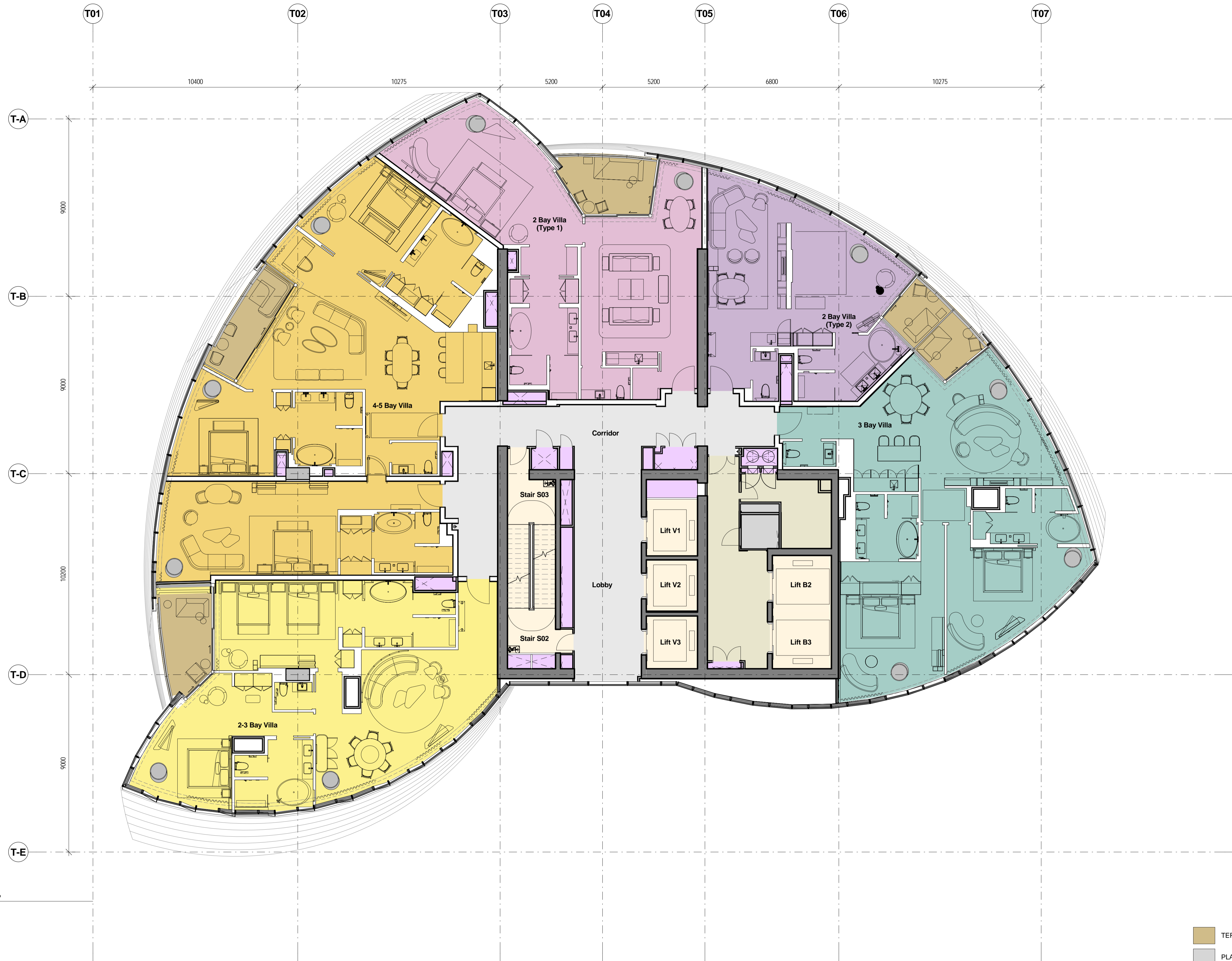
1 Level 30 FFL 1 : 100
