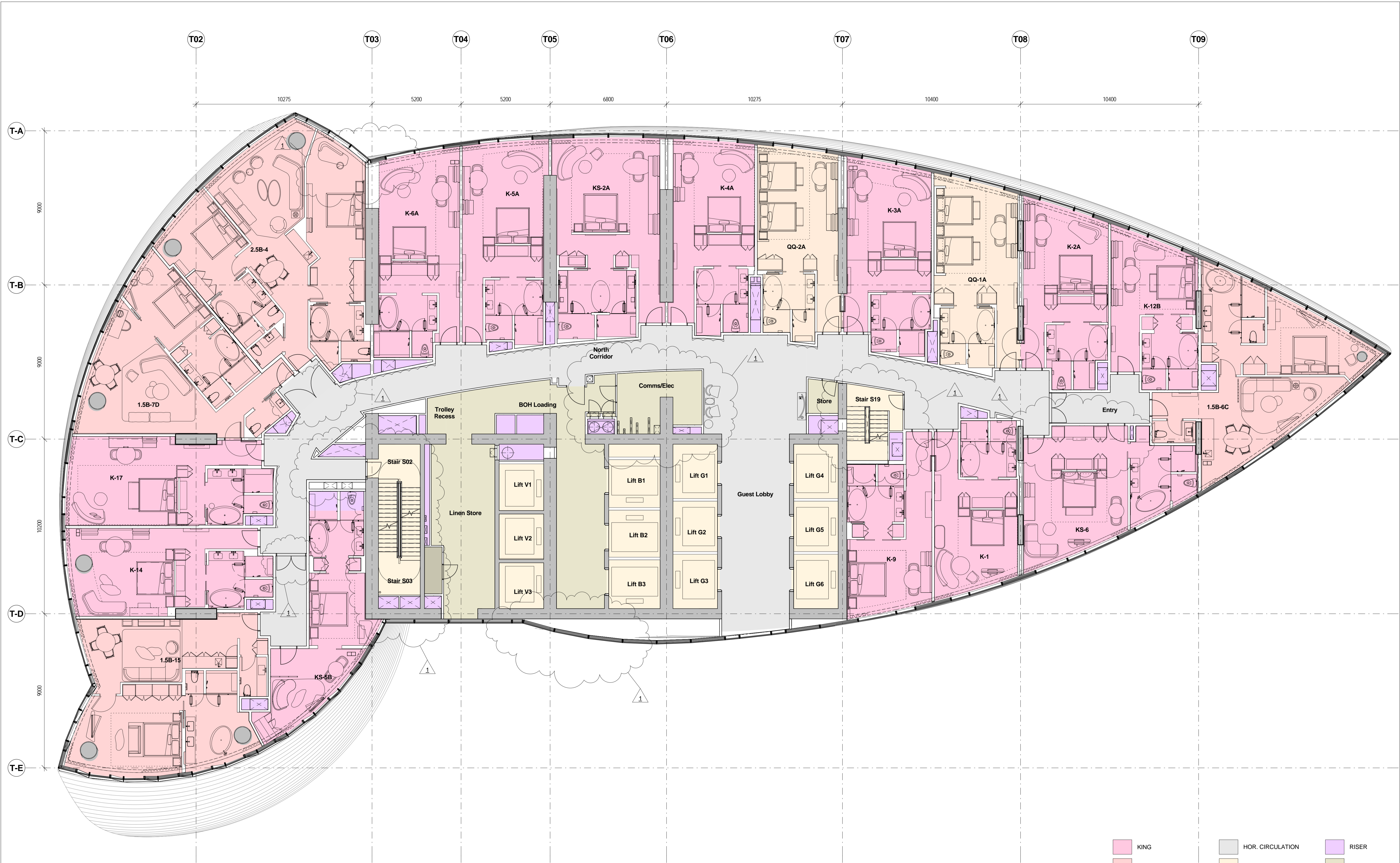
1 Level 22 FFL 1 : 100
