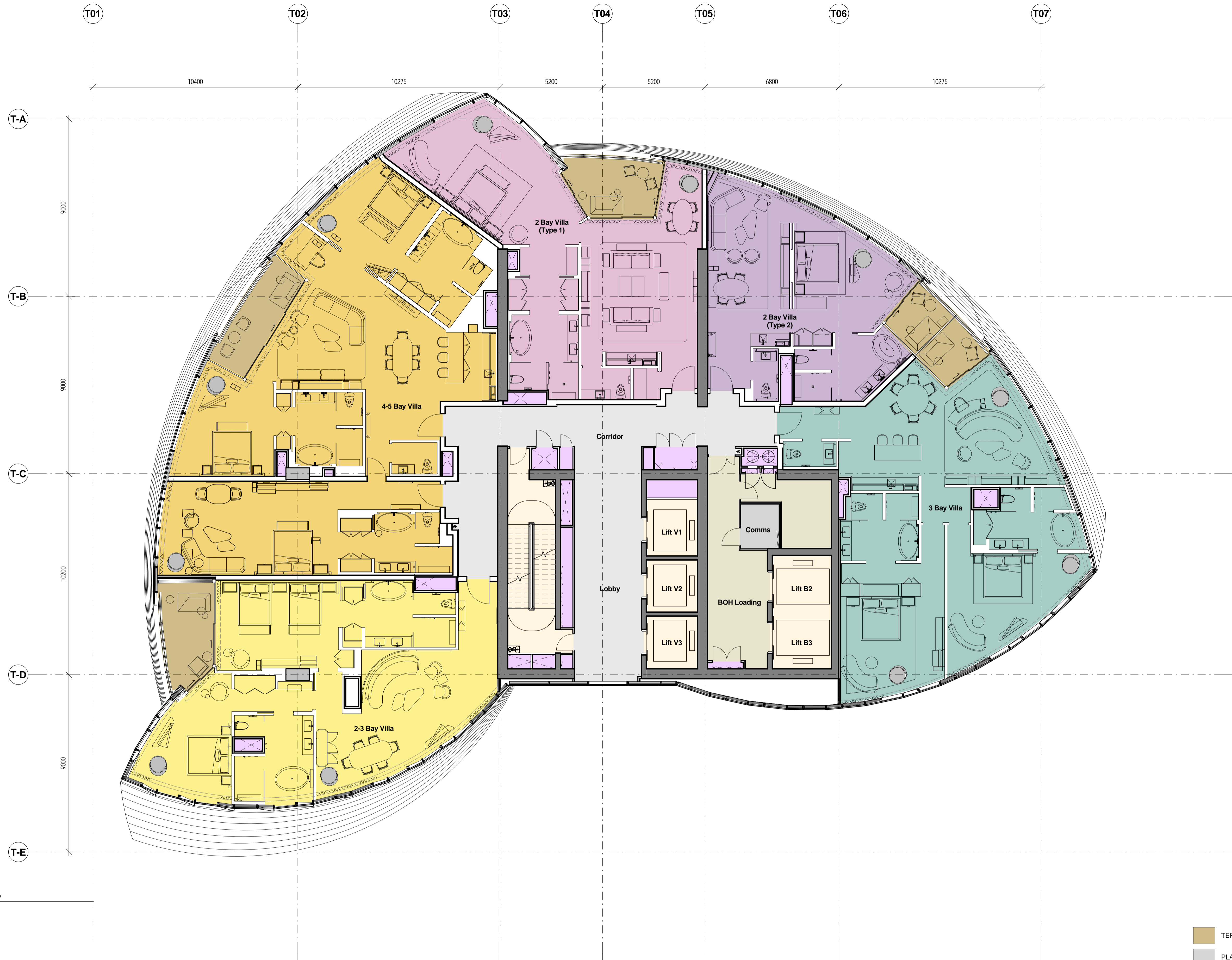
1 Level 31 FFL 1 : 100
