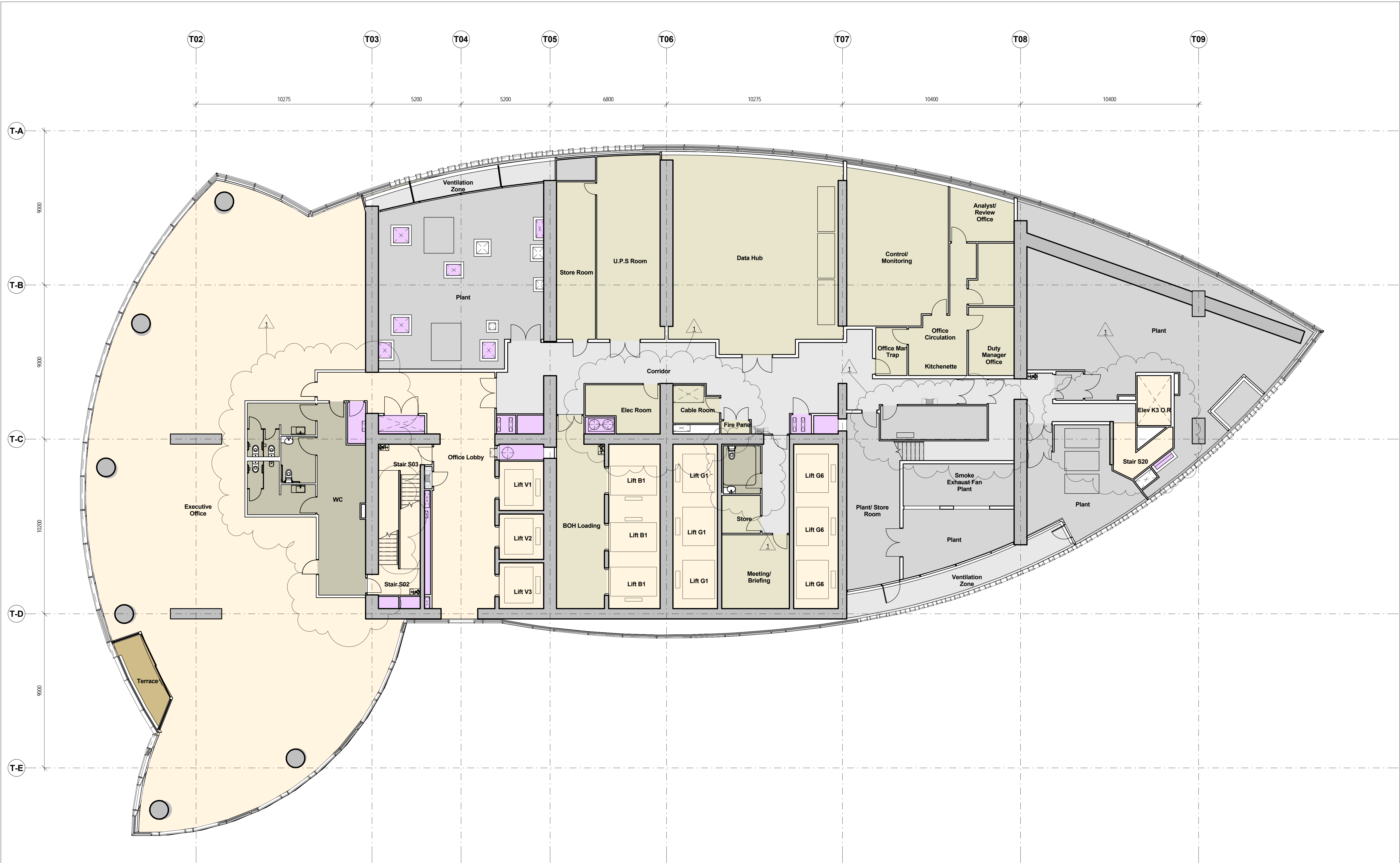
1 Level 05 FFL 1 : 100
