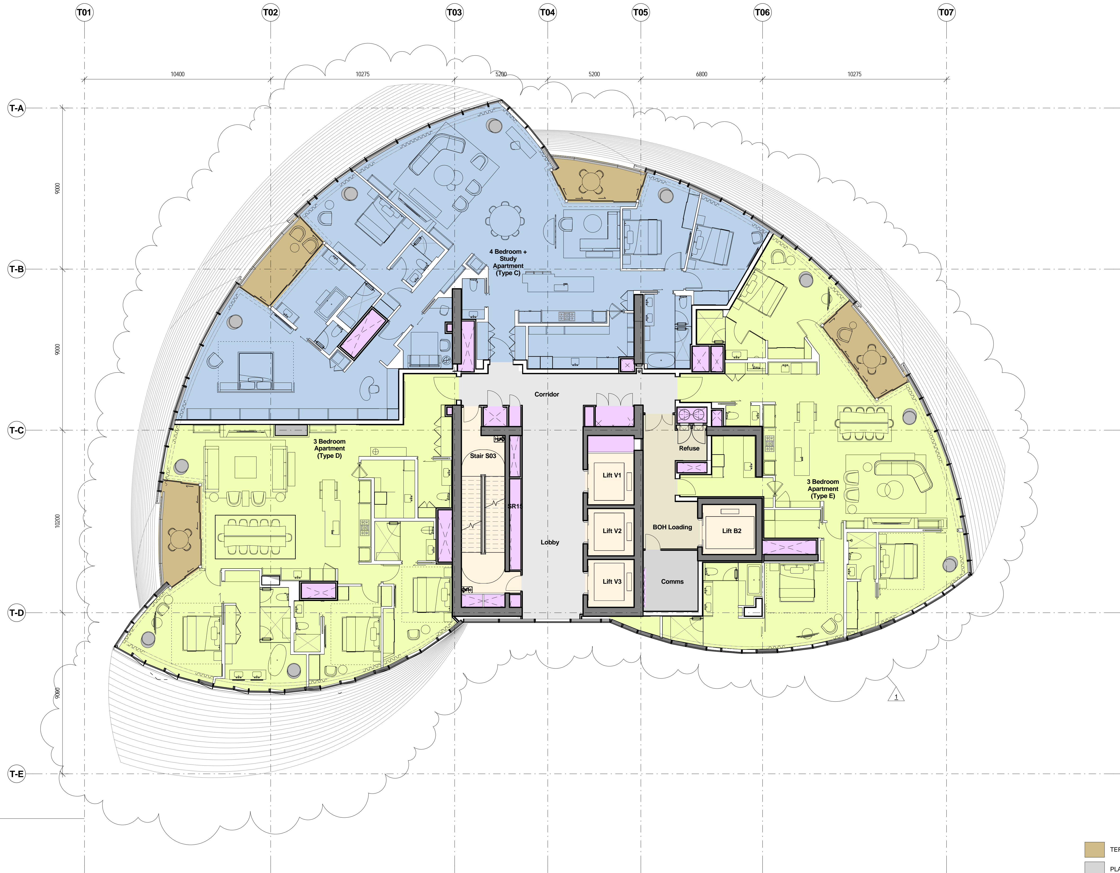
1 Level 40 1 : 100
