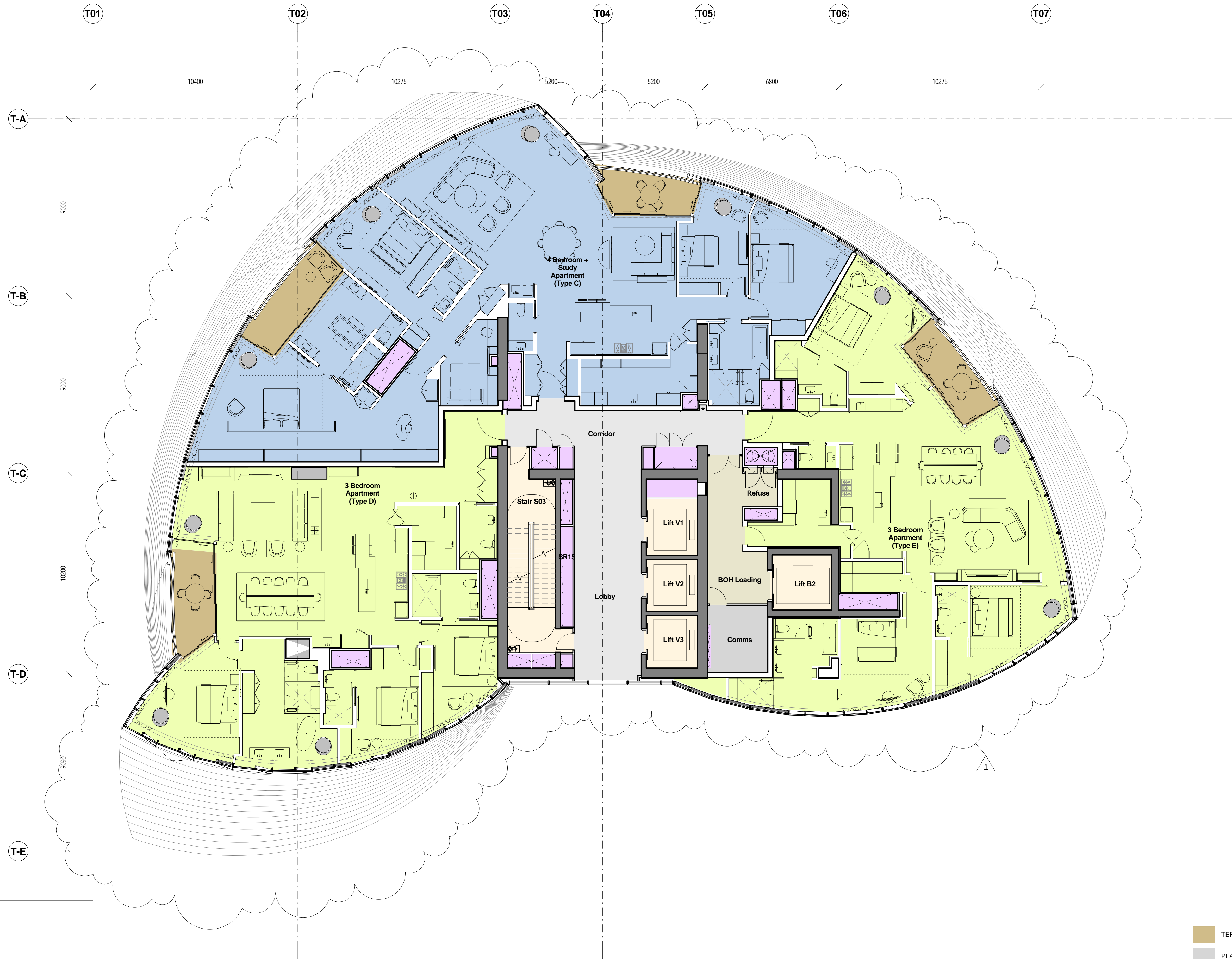
1 Level 38 1 : 100
