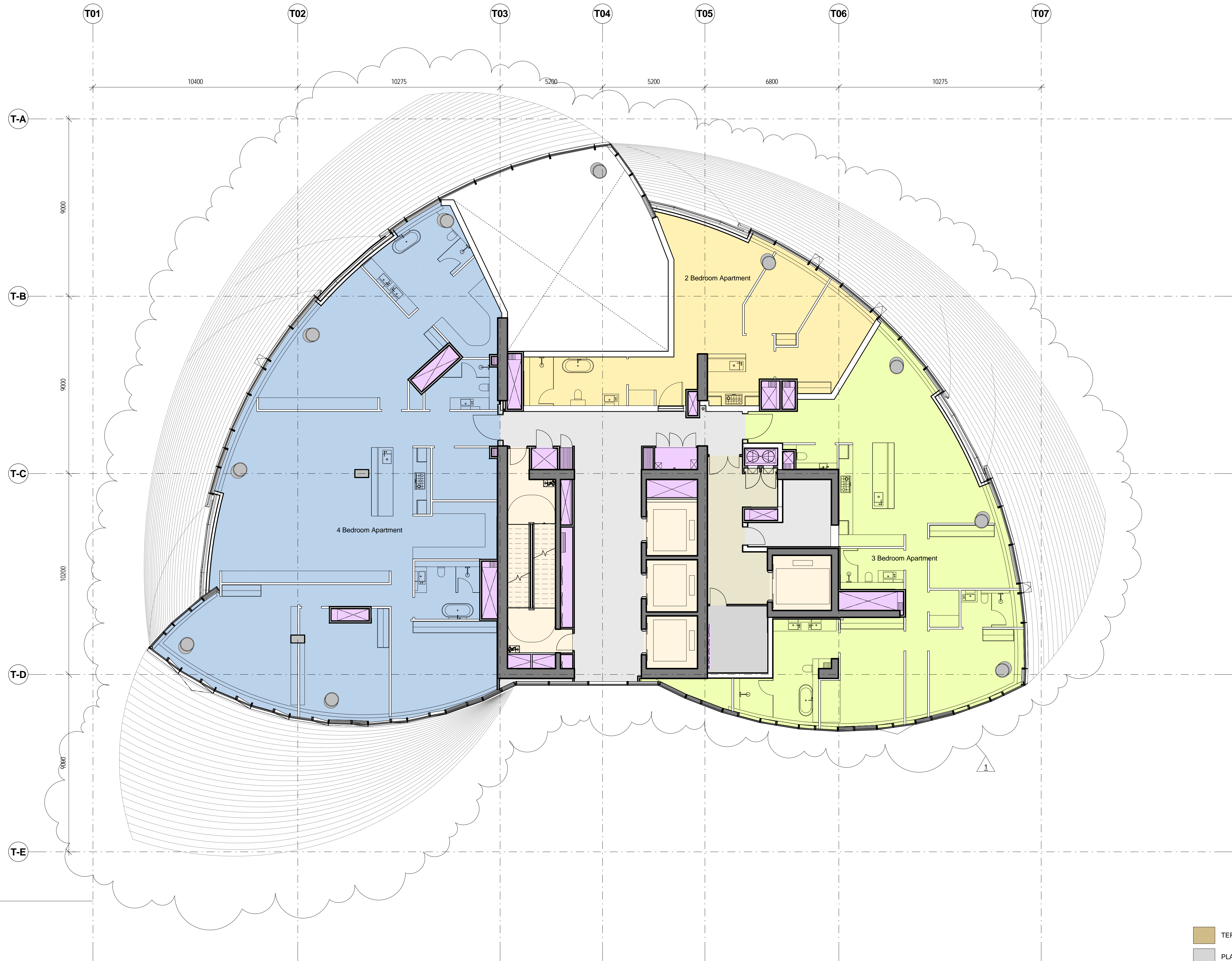
1 Level 49 1 : 100
