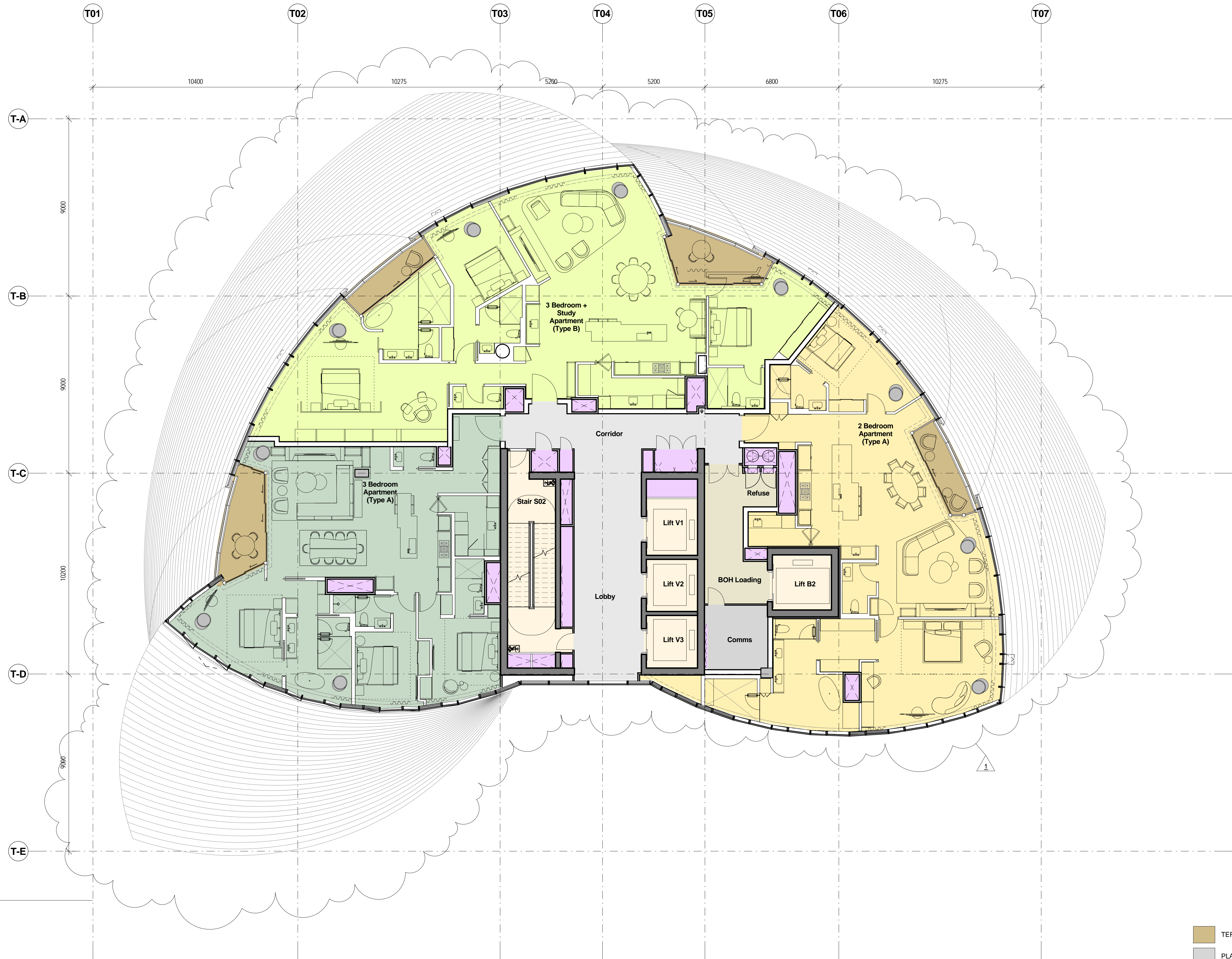
1 Level 53 1 : 100
