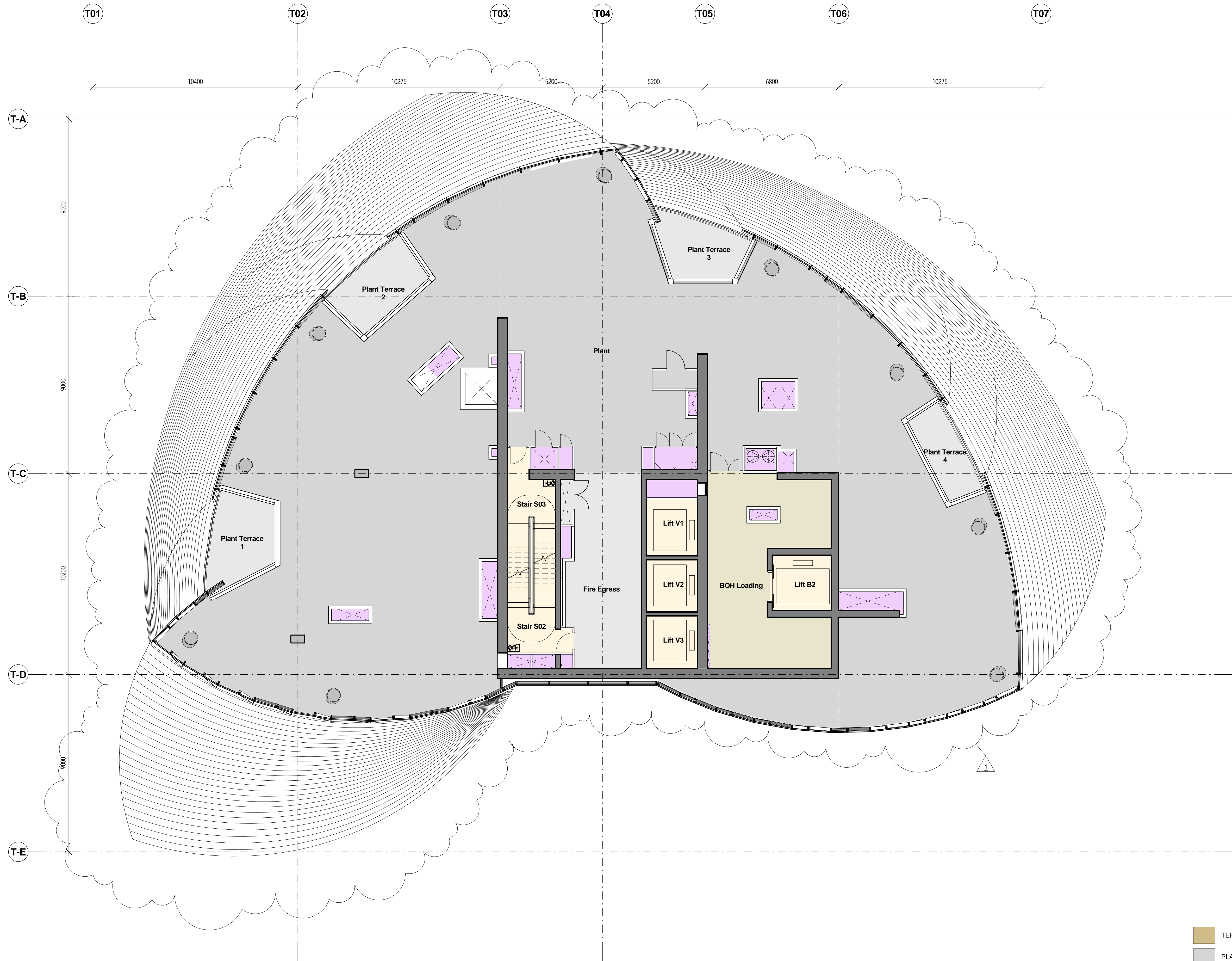
1 Level 50 1 : 100
