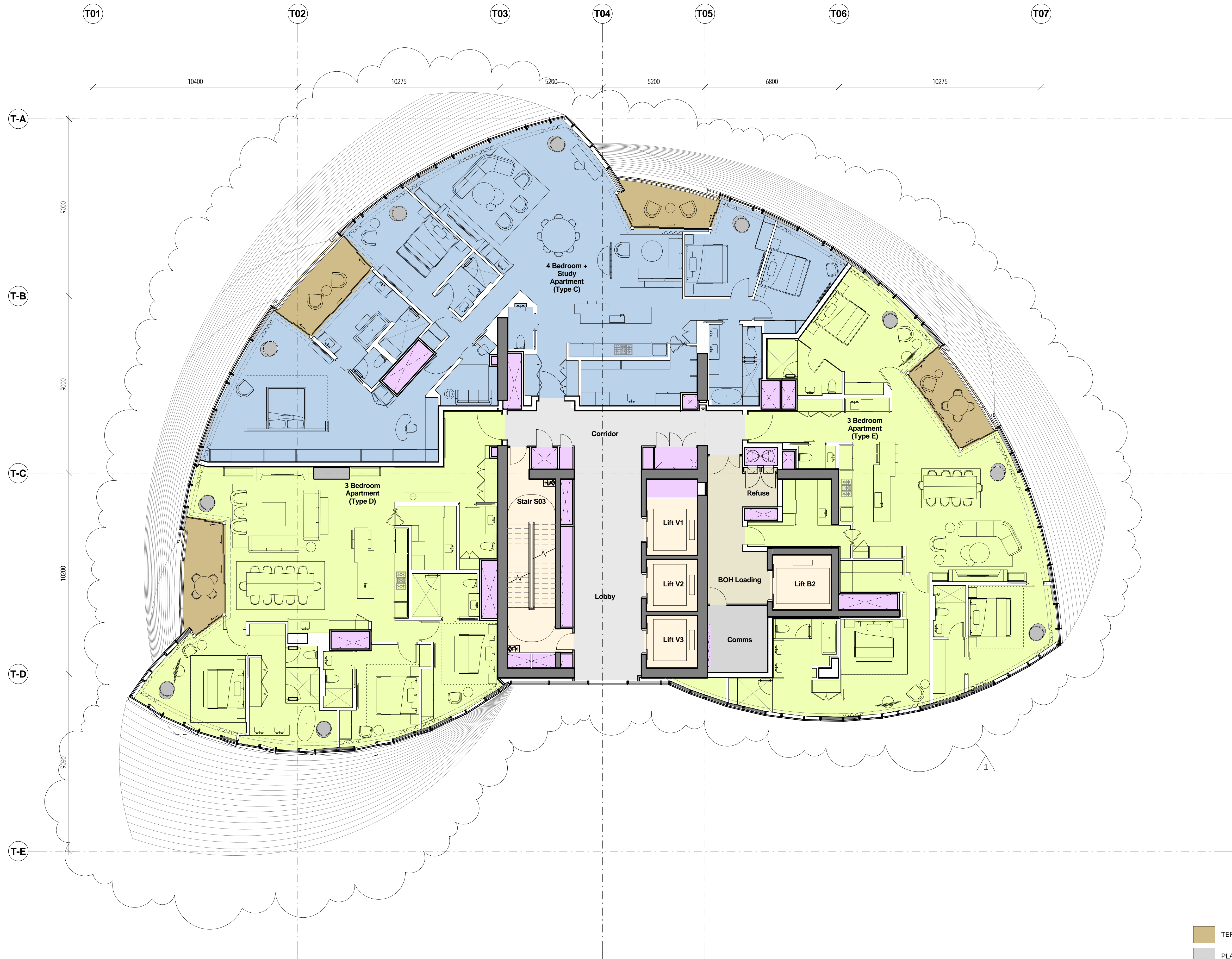
1 Level 42 1 : 100
