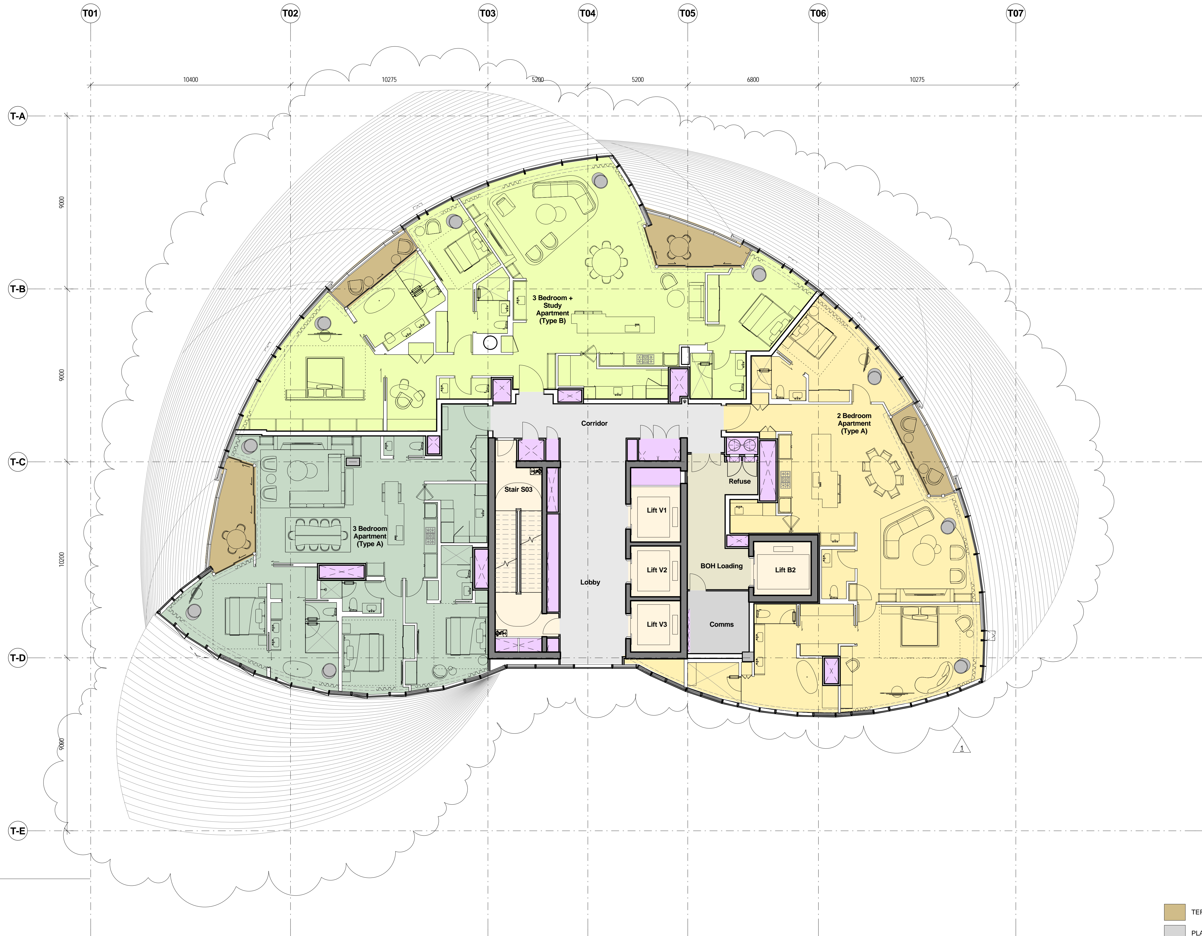
1 Level 52 1 : 100
