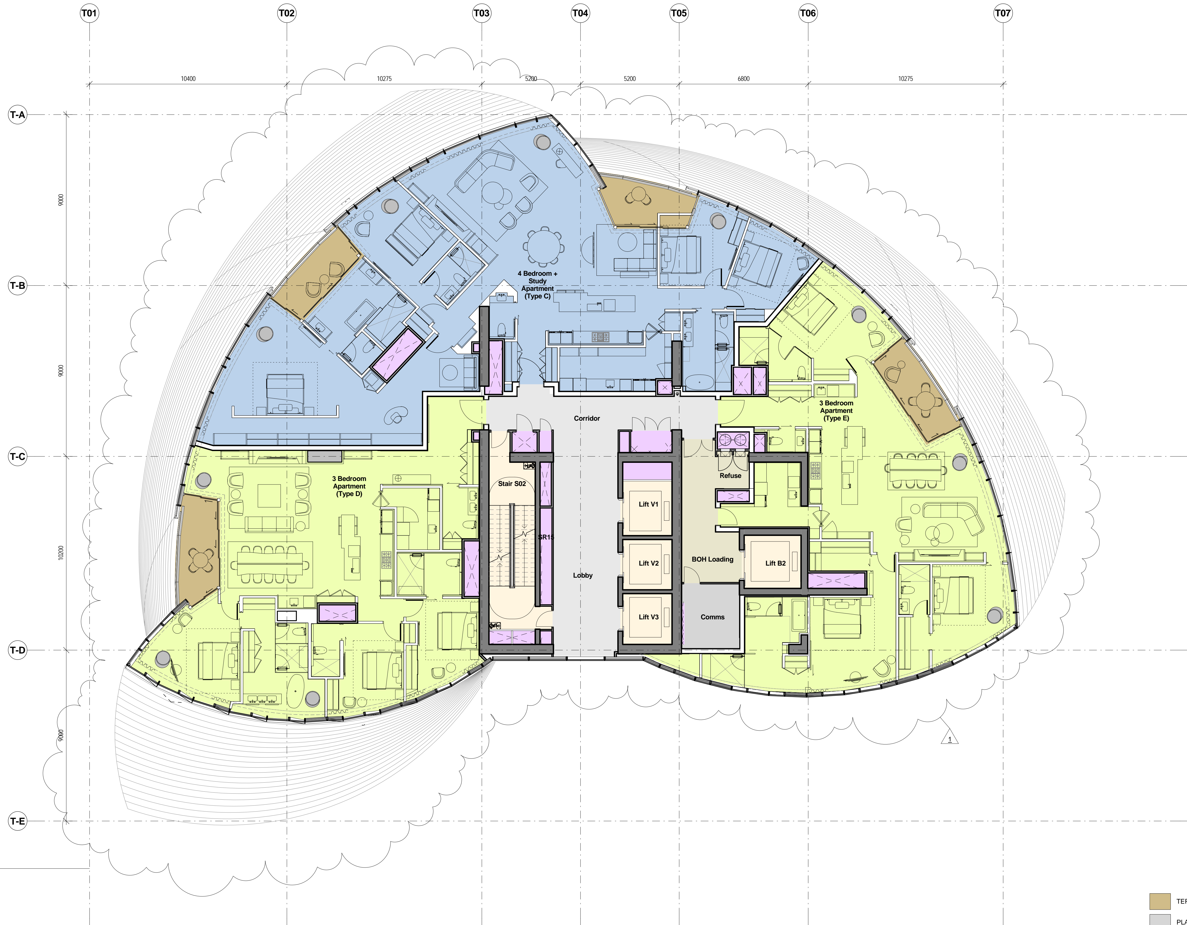
1 Level 43 1 : 100
