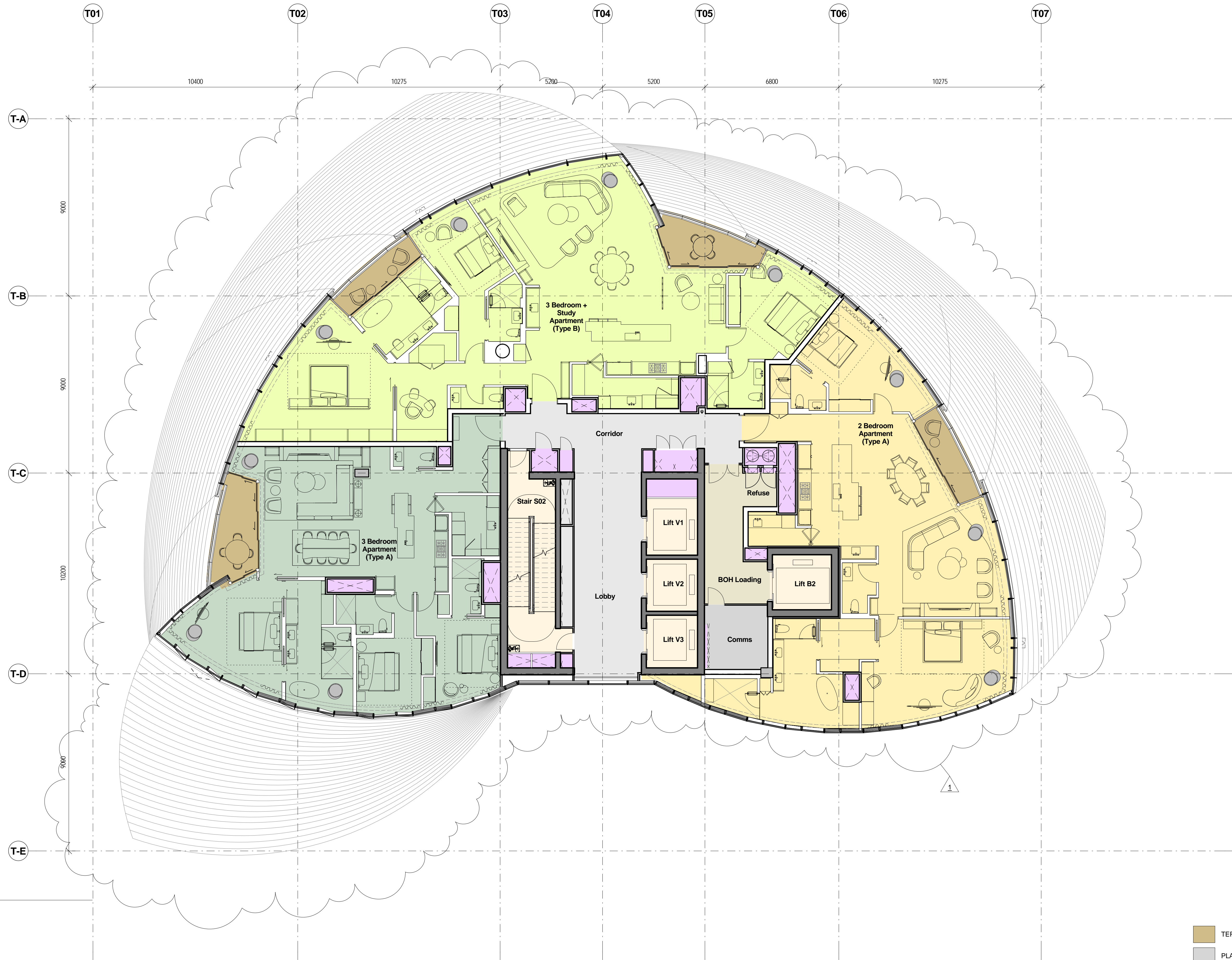
1 Level 51 1 : 100
