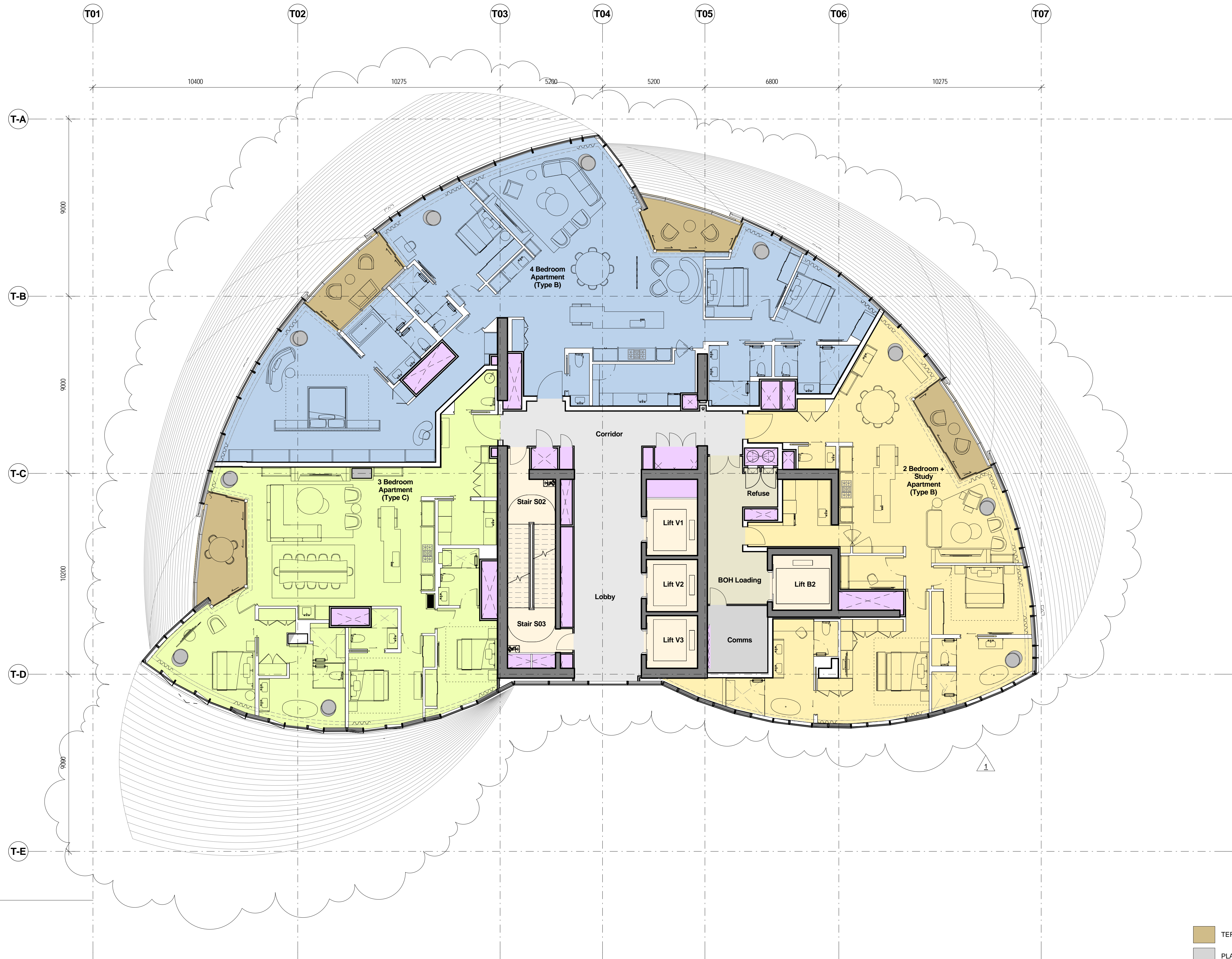
1 Level 47 1 : 100
