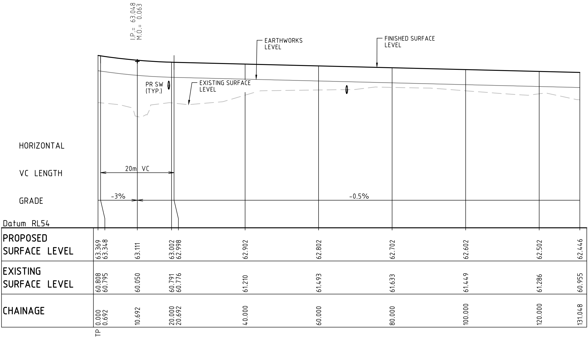
ROAD 05 LONGITUDINAL SECTION
