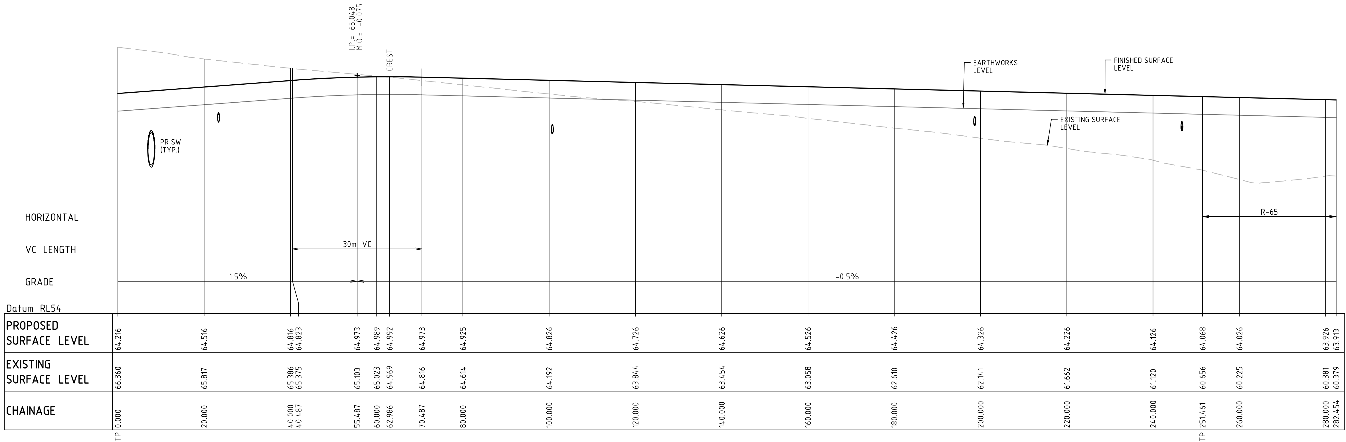
ROAD 04 LONGITUDINAL SECTION SCALE 1:500 HORI. 1:100 VERT.
