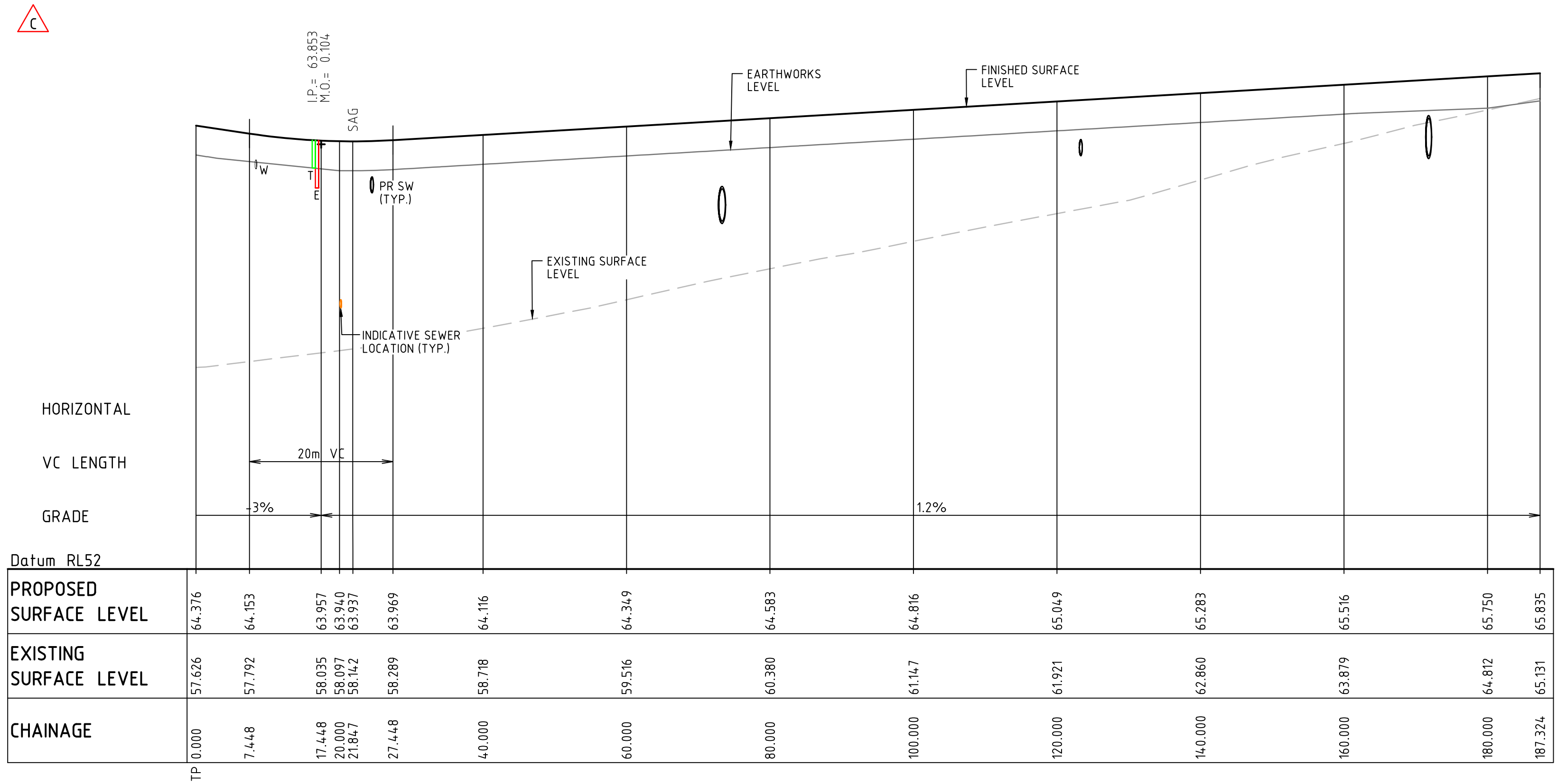
ROAD 02 LONGITUDINAL SECTION
