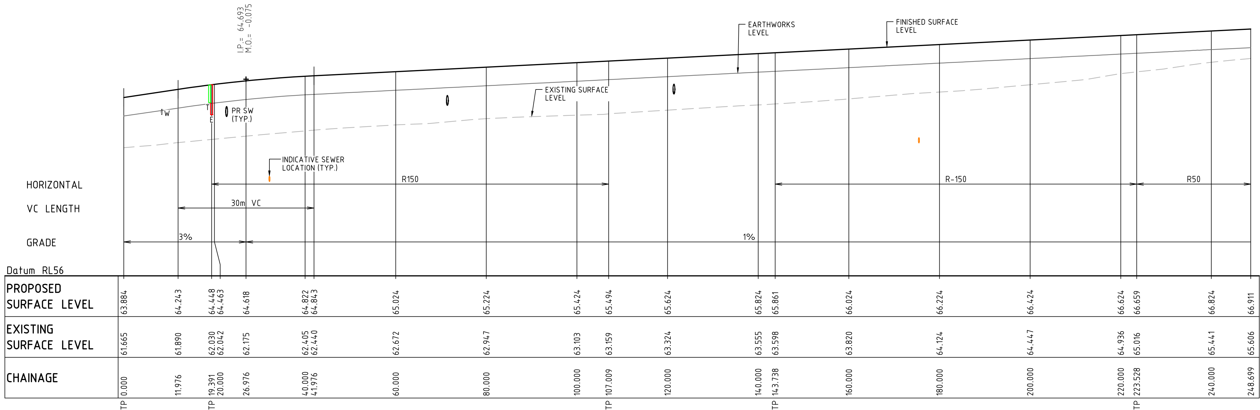
ROAD 03 LONGITUDINAL SECTION SCALE 1:500 HORI.
