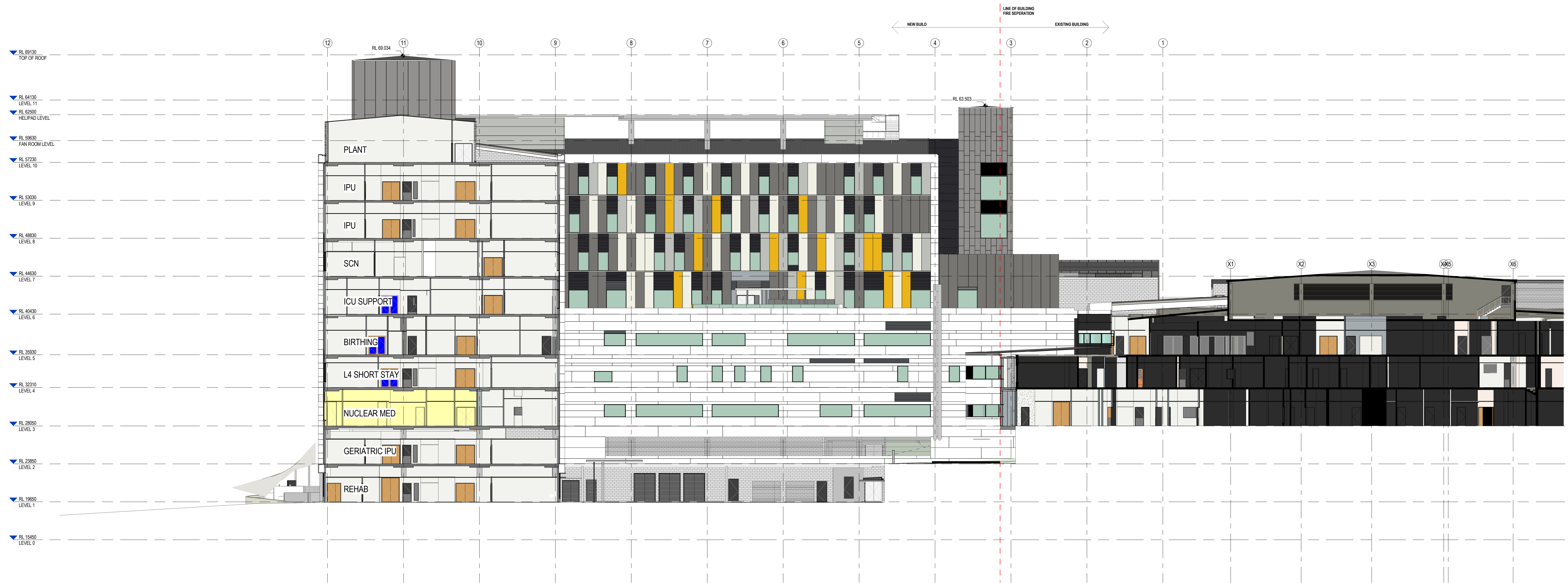
1 Section 96 - I-I
