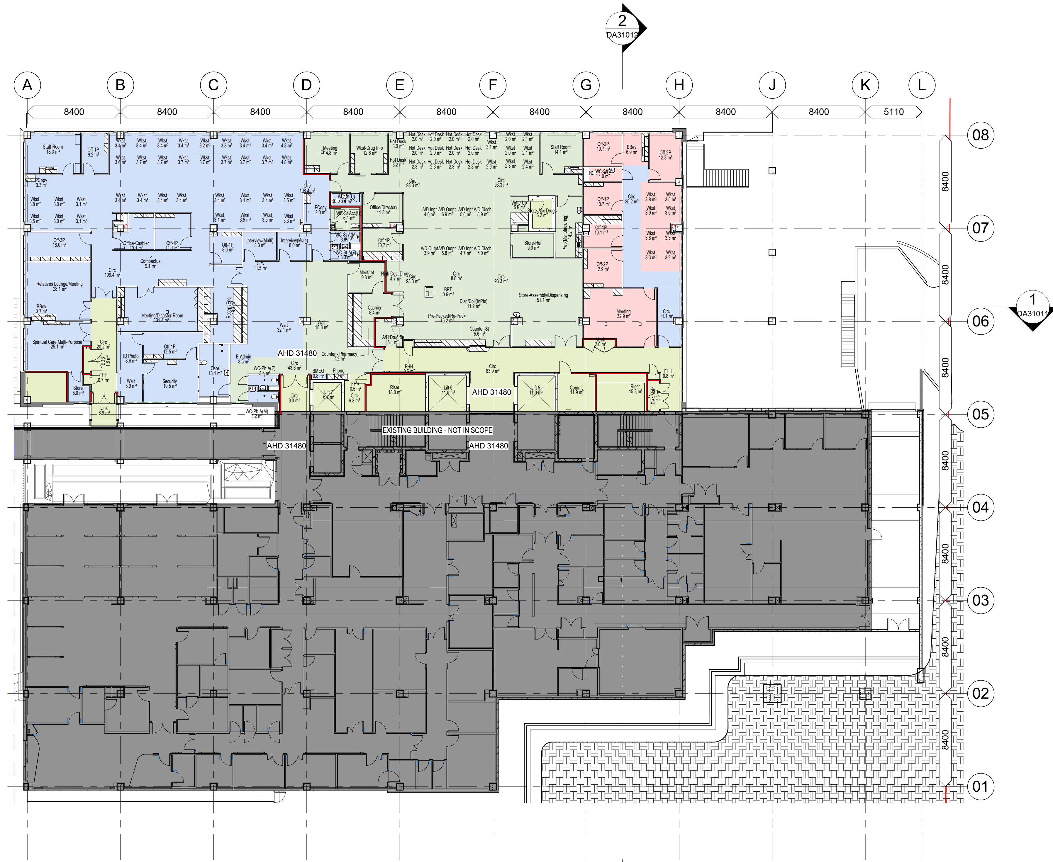
1 GA - Level 04 3B2 A30001 1 : 200
