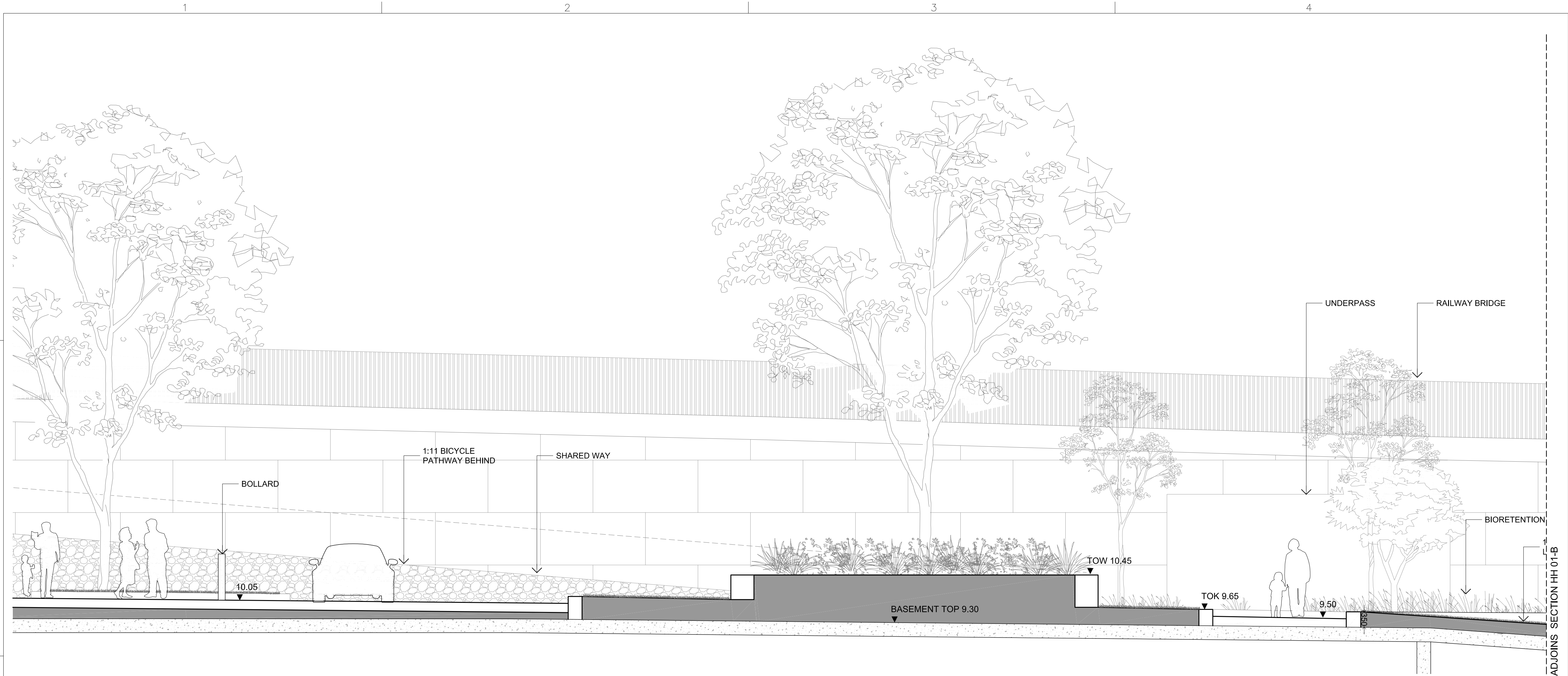
1 SECTION HH 01-A SCALE - 1:50 @ A1 1:200 @A3
