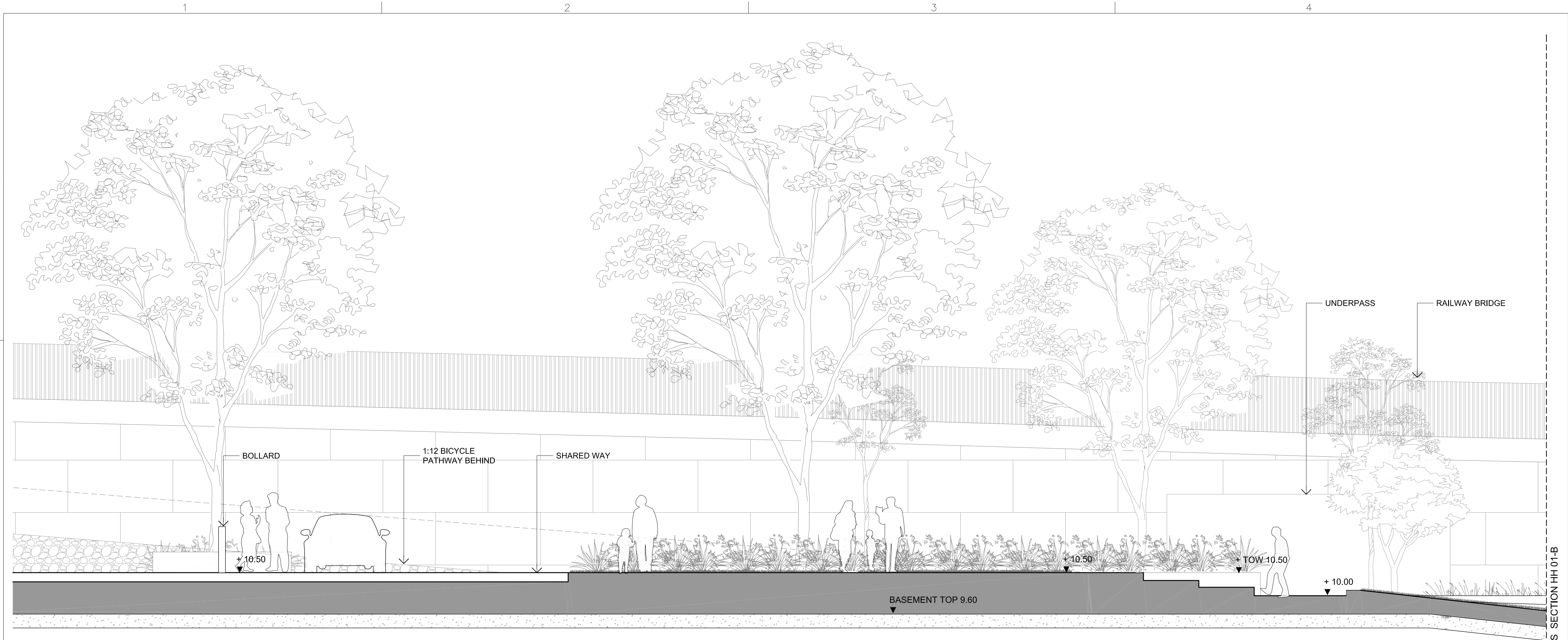
1 SECTION HH 01-A SCALE - 1:50 @ A1 1:200 @A3
