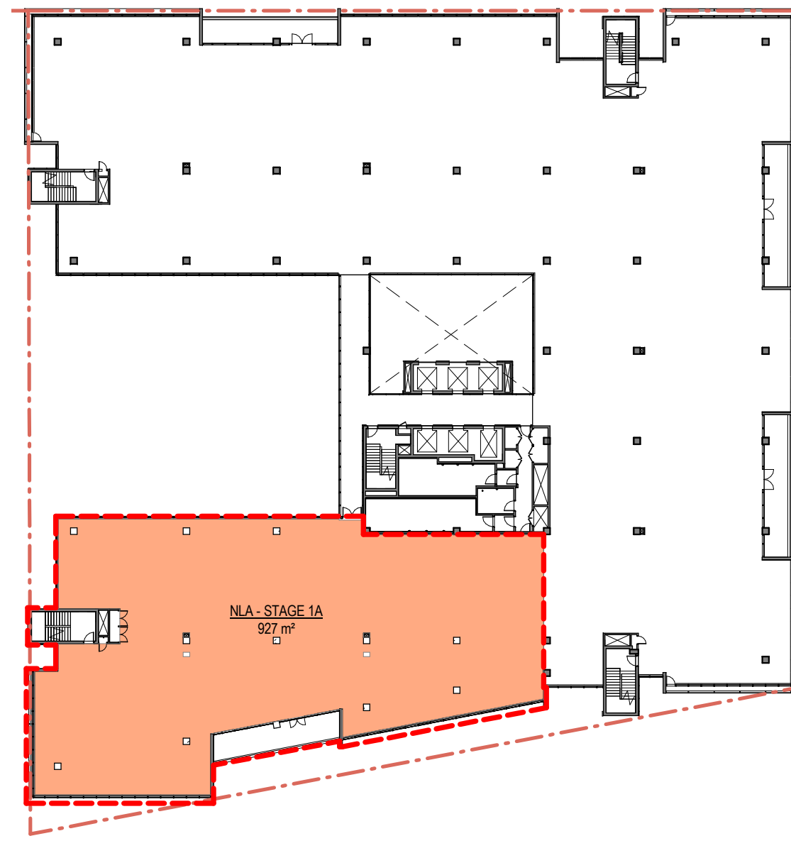
8 Level 7 1 : 500
