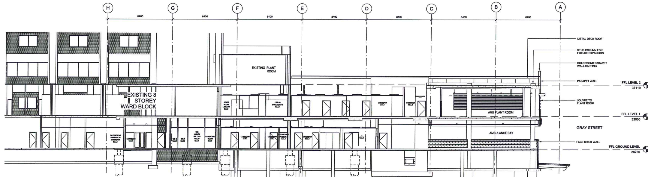
2 SECTION 01 1:100
