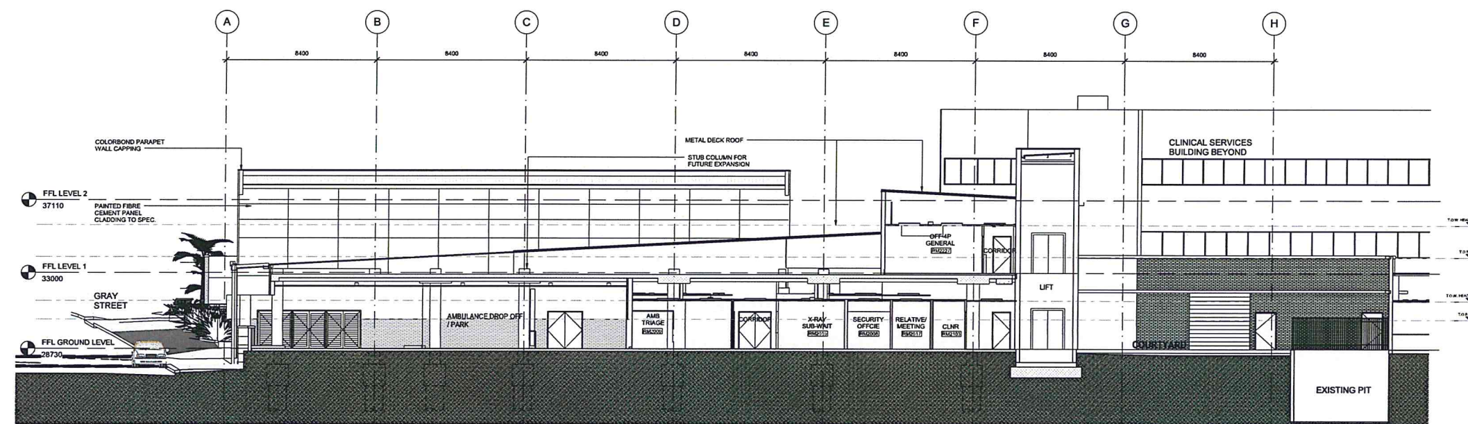
1 SECTION 02 1:100
