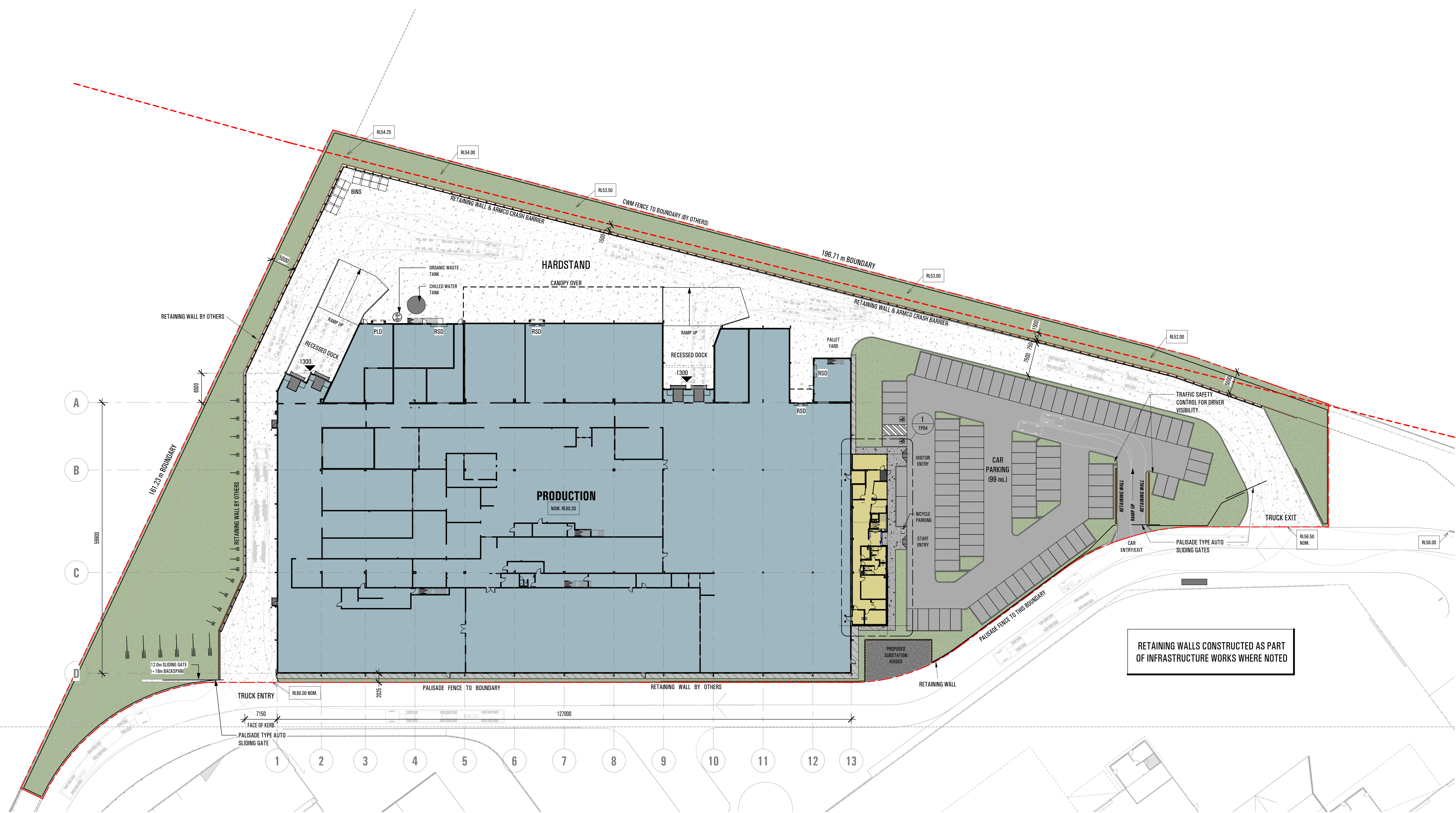
1 SITE PLAN 1 : 400
