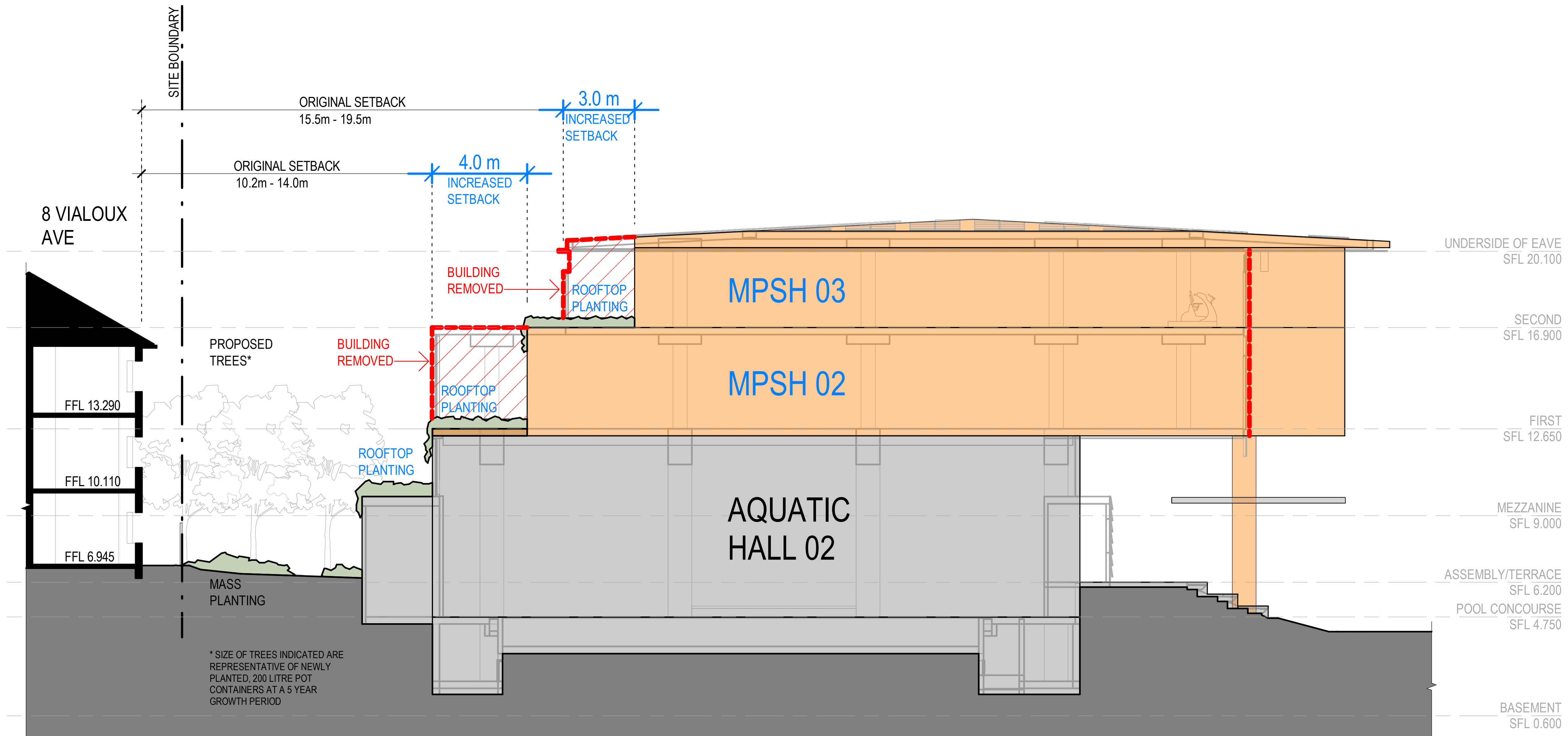
SECTION 01
