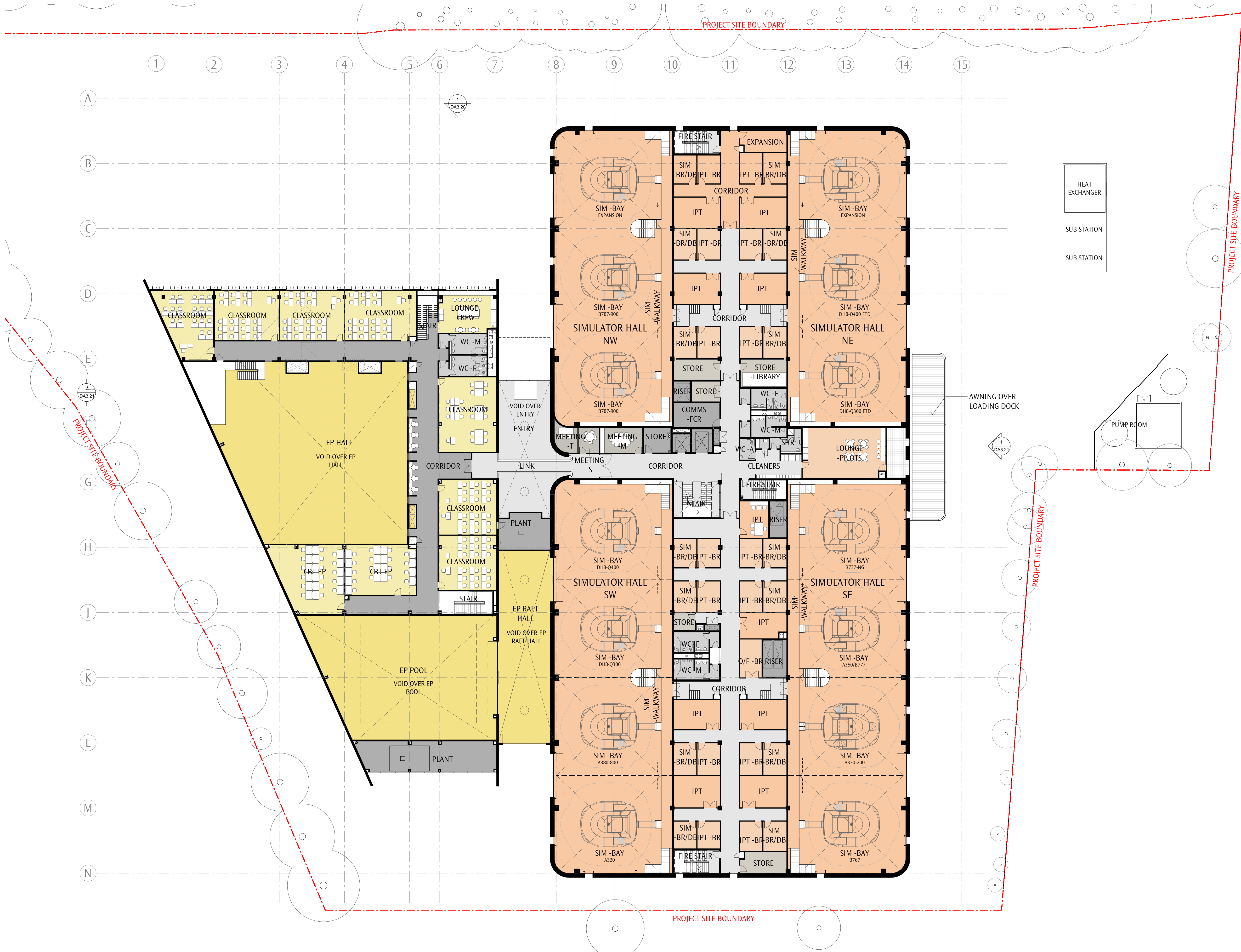
1 PLAN - L01 1 : 250
