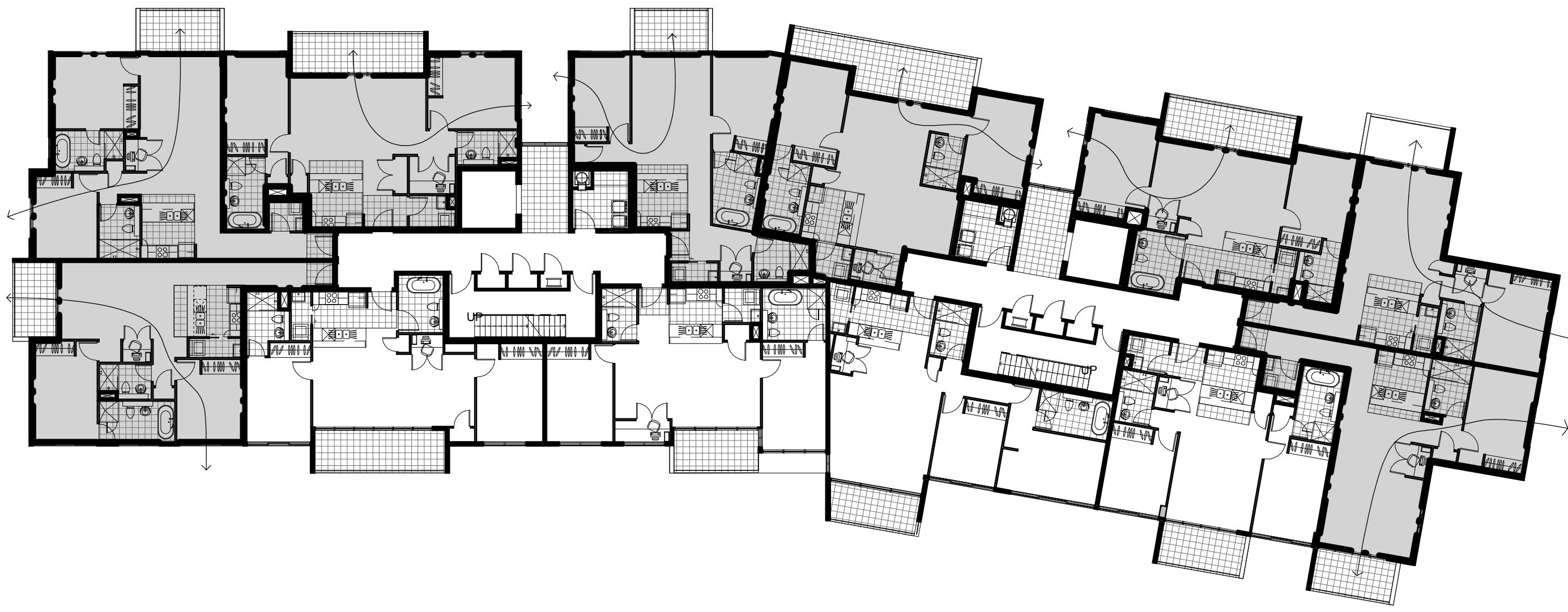
3 CV LEVEL 2 1 : 200
