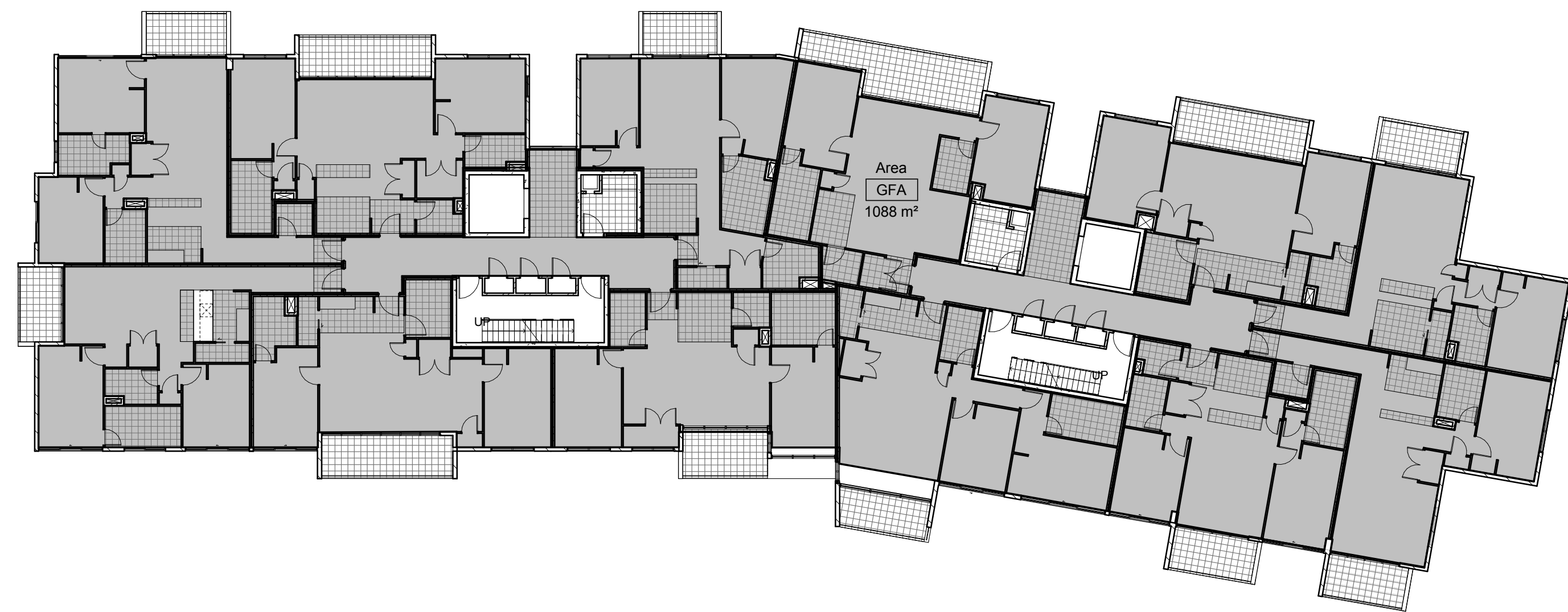
2 LEVEL 1 1 : 200
