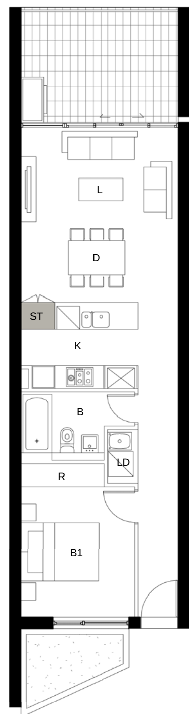
3 DETAIL PLAN BLDG D - Apartment Type 3 1 BED - 53sqm Storage 1.7cbm D.1.03 D.2.05 D.4.04 D.6.03 D.1.04 D.3.03 D.4.05 D.6.04 D.1.05 D.3.04 D.5.03 D.6.05 D.2.03 D.3.05 D.5.04 D.2.04 D.4.03 D.5.05
