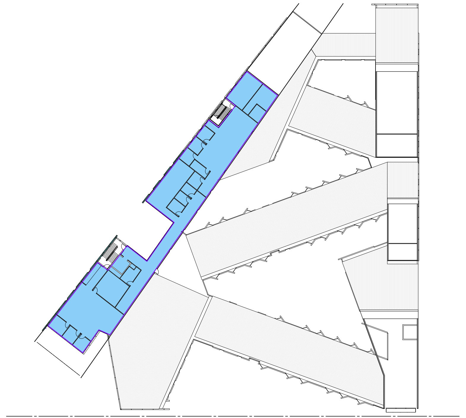
3 LEVEL 03 1 : 500
