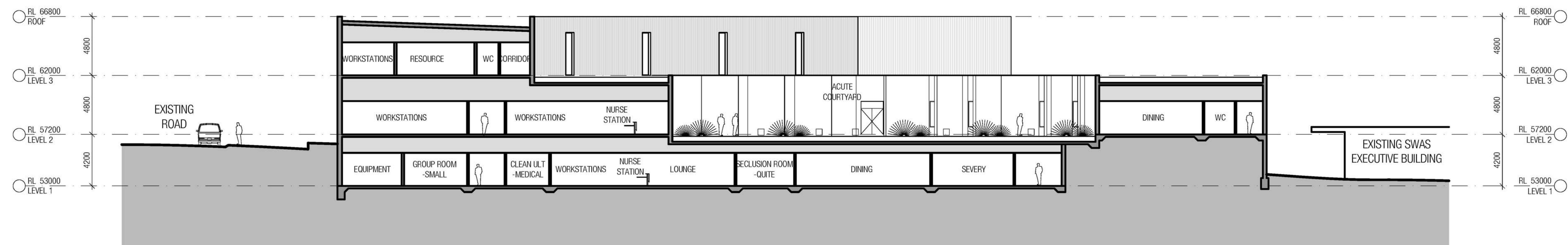
1 SECTION 1 1 : 200
