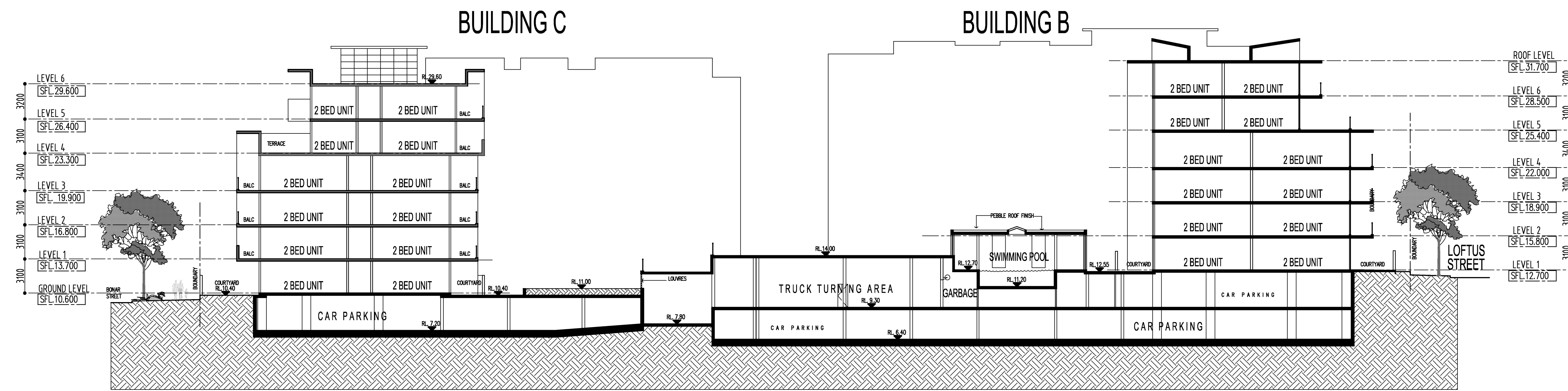
SECTION A-A
