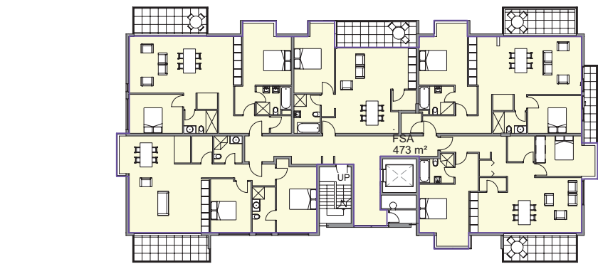
6 Level 4 1 : 200
