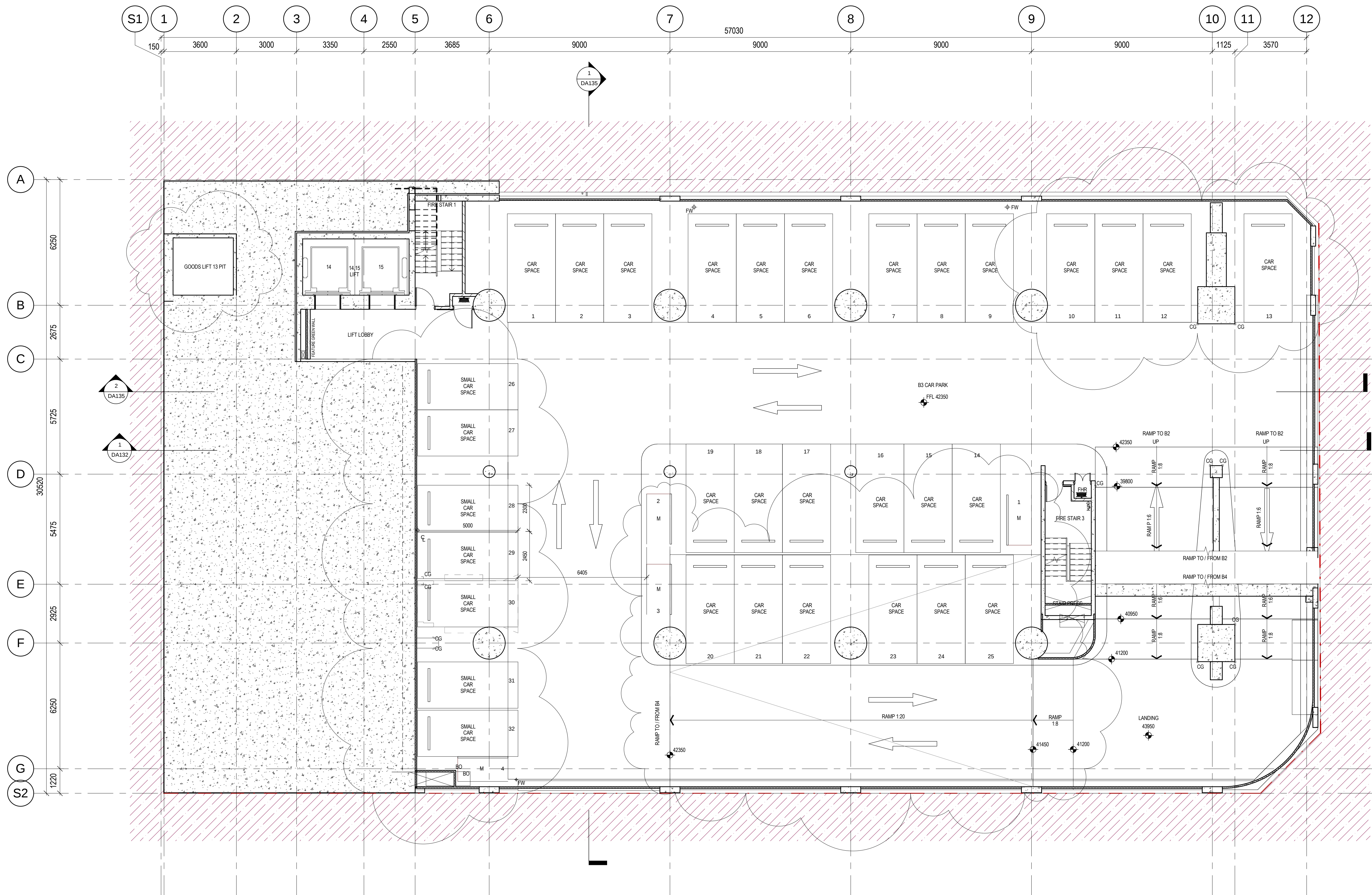
1 Level B3 SCALE: 1 : 100
