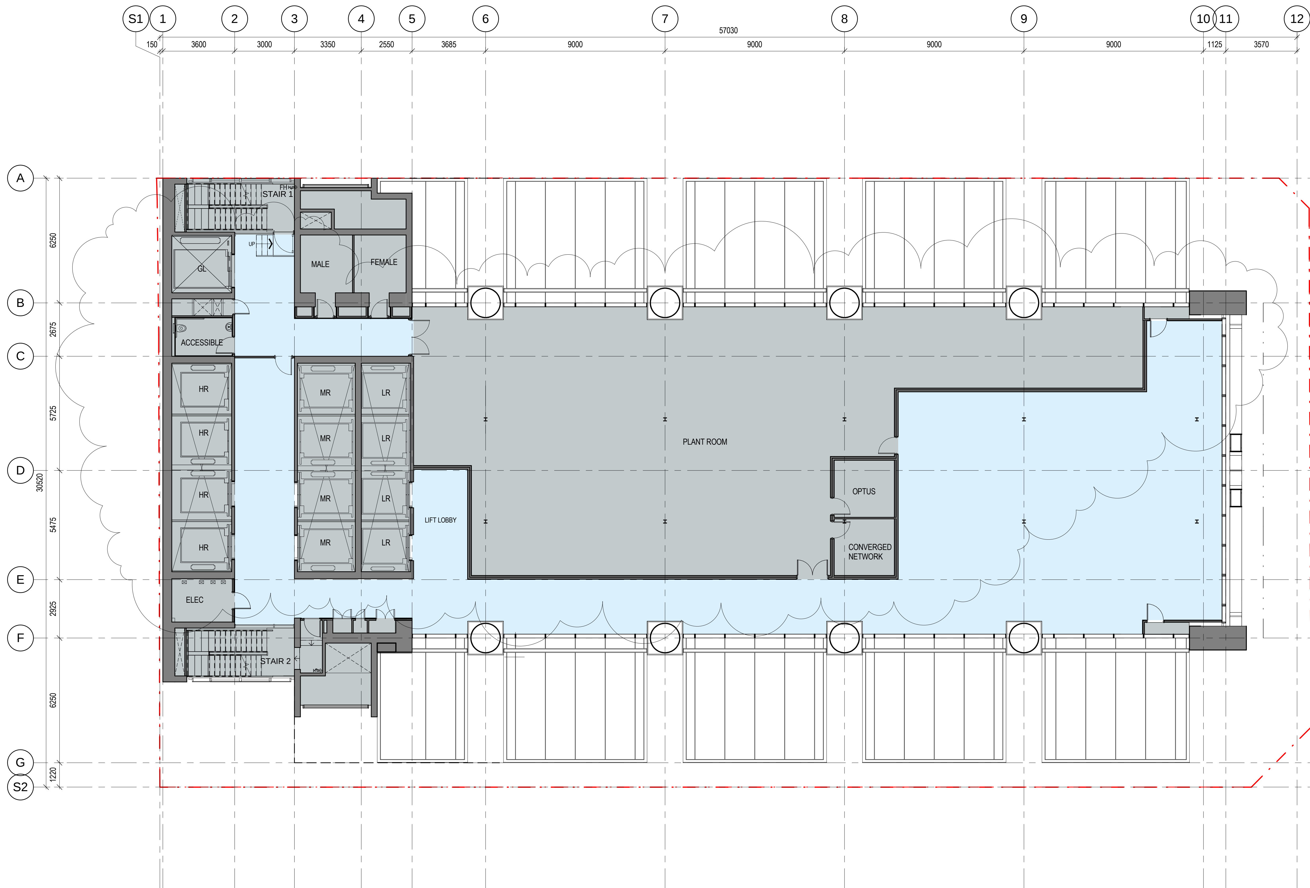
1 Level 1 Plan SCALE: 1 : 100
