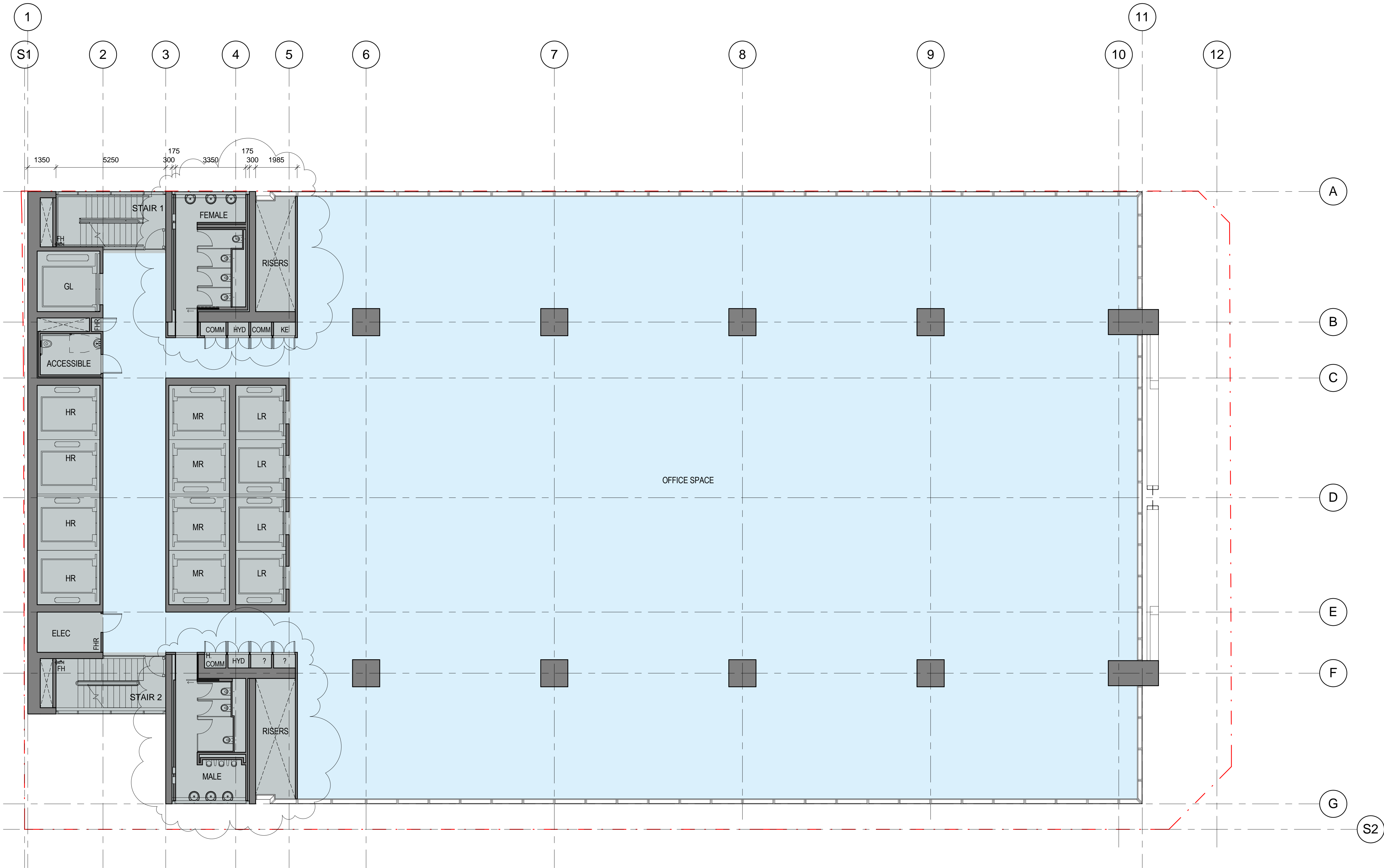
1 Typ. Low Rise 1 : 100
