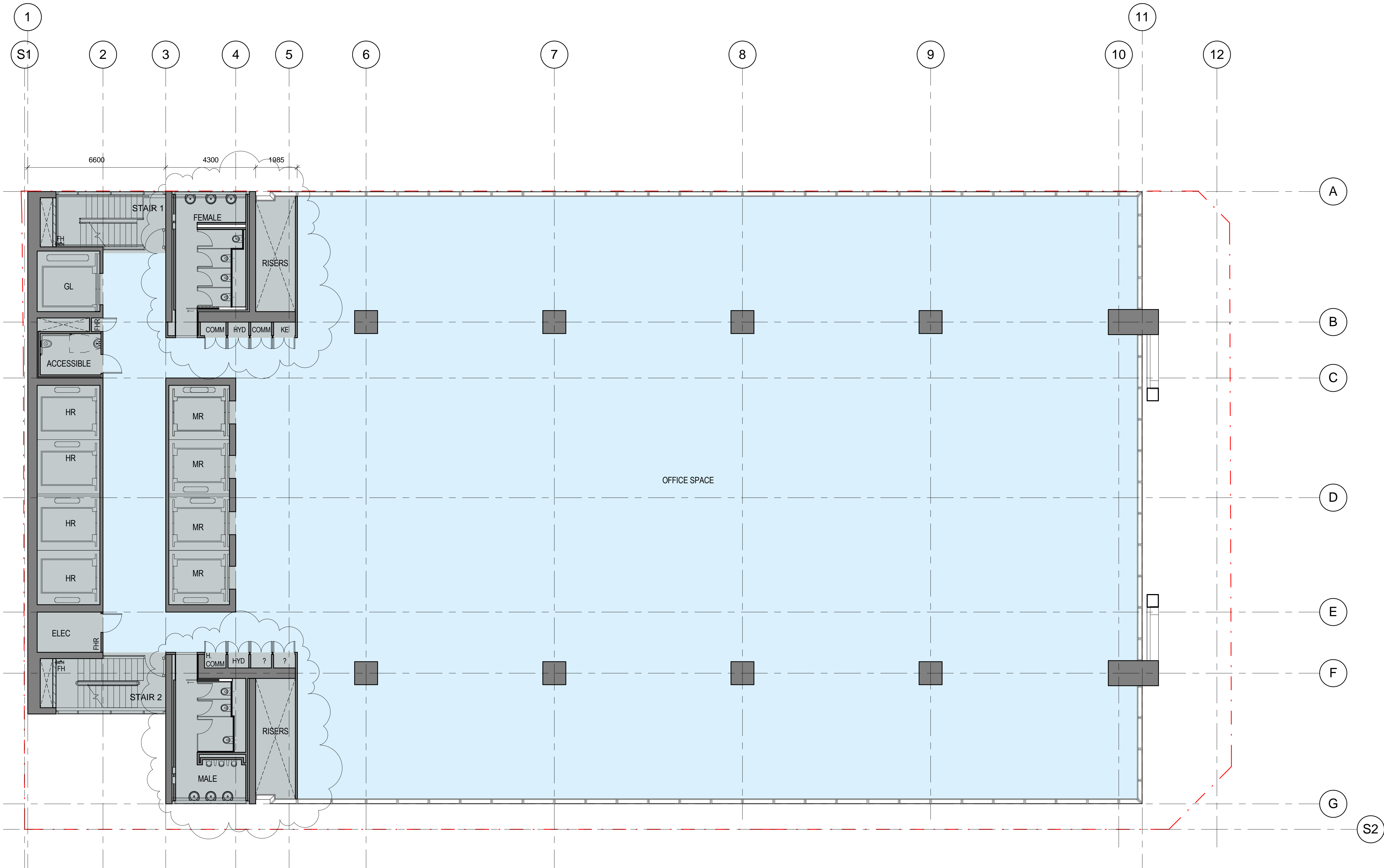
1 Typ. Mid Rise 1 : 100
