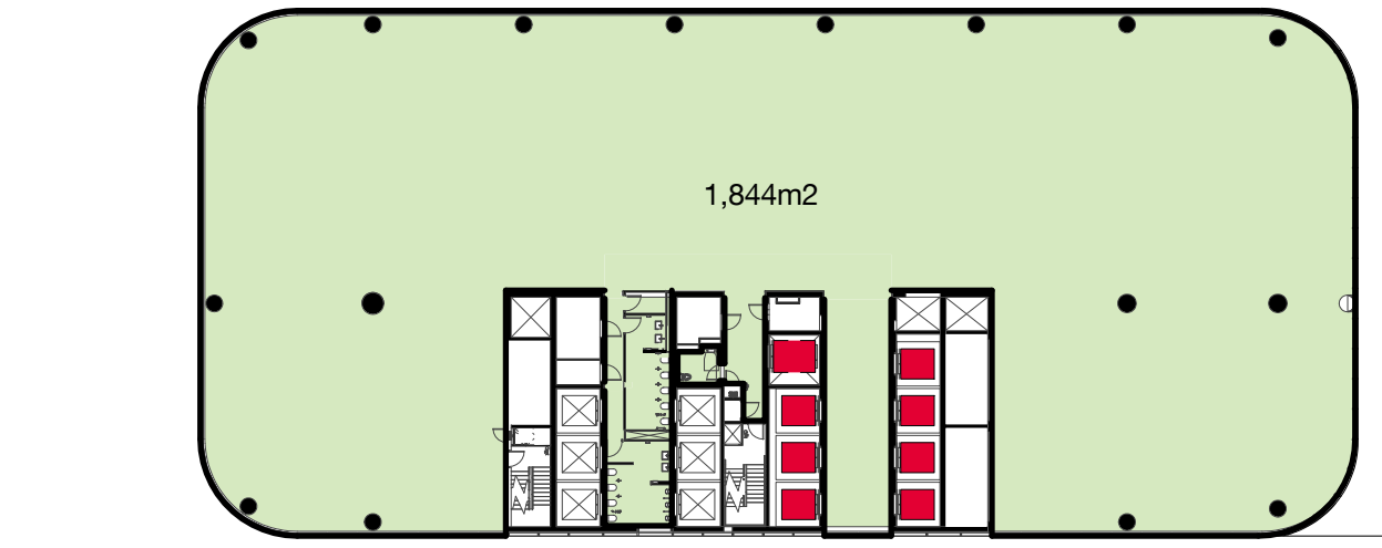
2 GFA - Level 19 1 : 500
