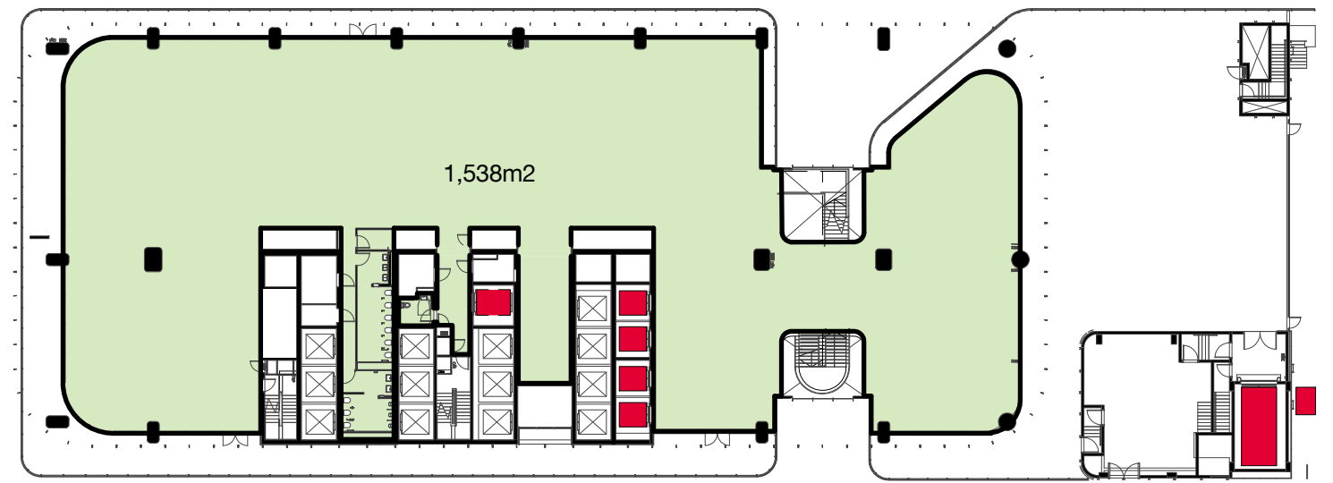
9 GFA - Level 02 1 : 500
