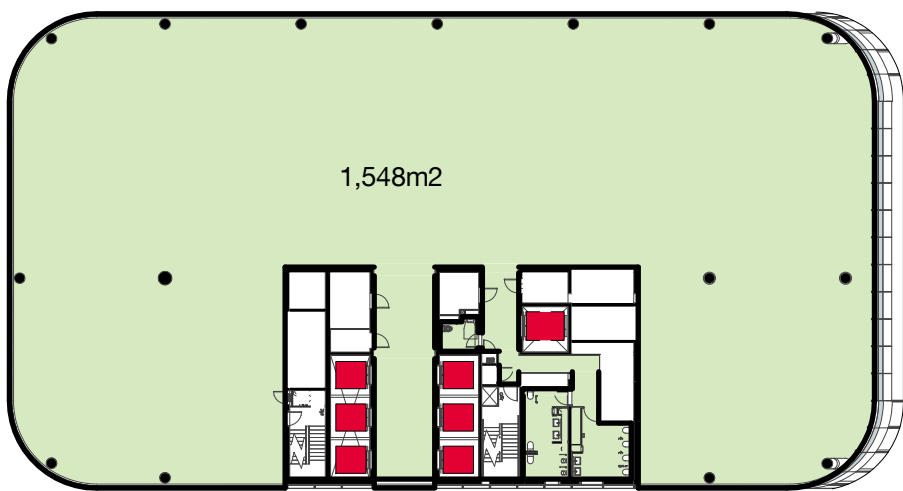
3 GFA - Level 32 1 : 500
