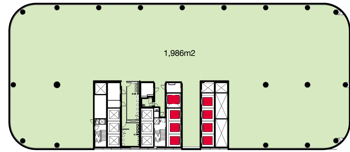
9 GFA - Level 14 1 : 500
