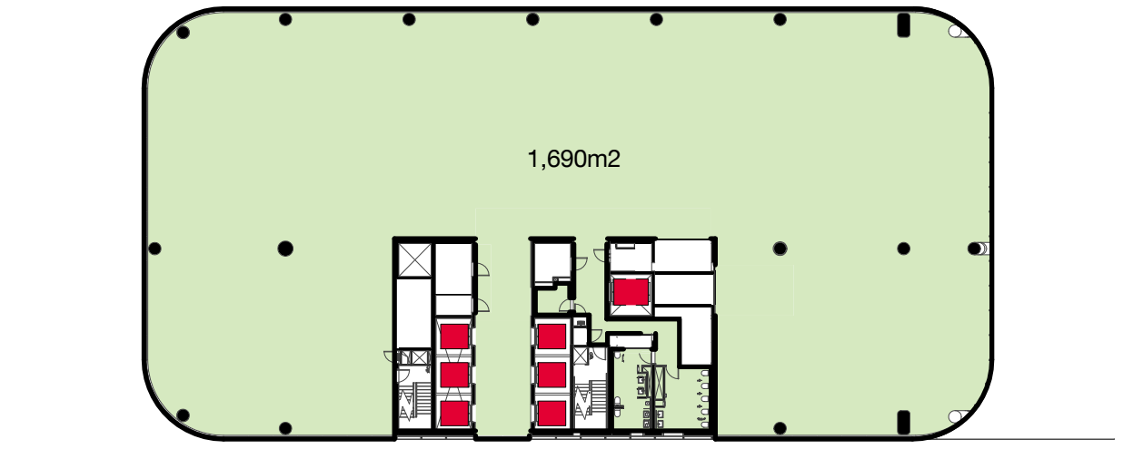
10 GFA - Level 27 1 : 500
