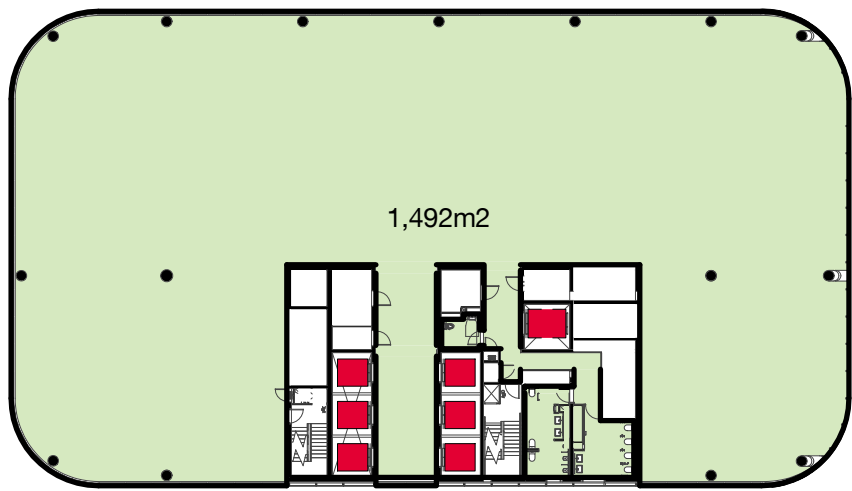
5 GFA - Level 34 1 : 500
