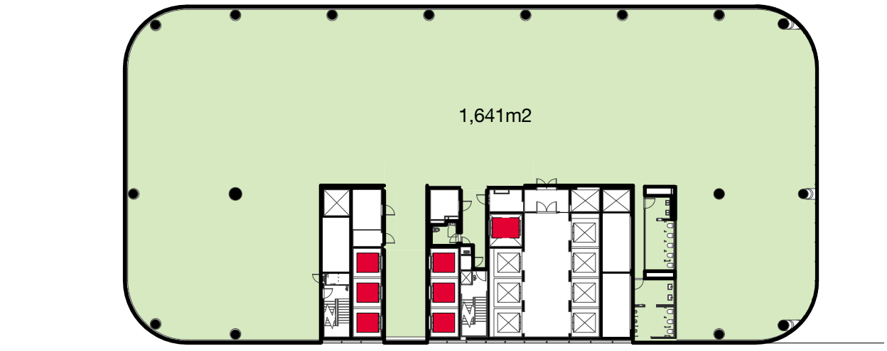
7 GFA - Level 24 1 : 500
