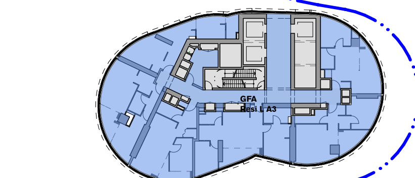
LEVEL 10 A3 1:500
