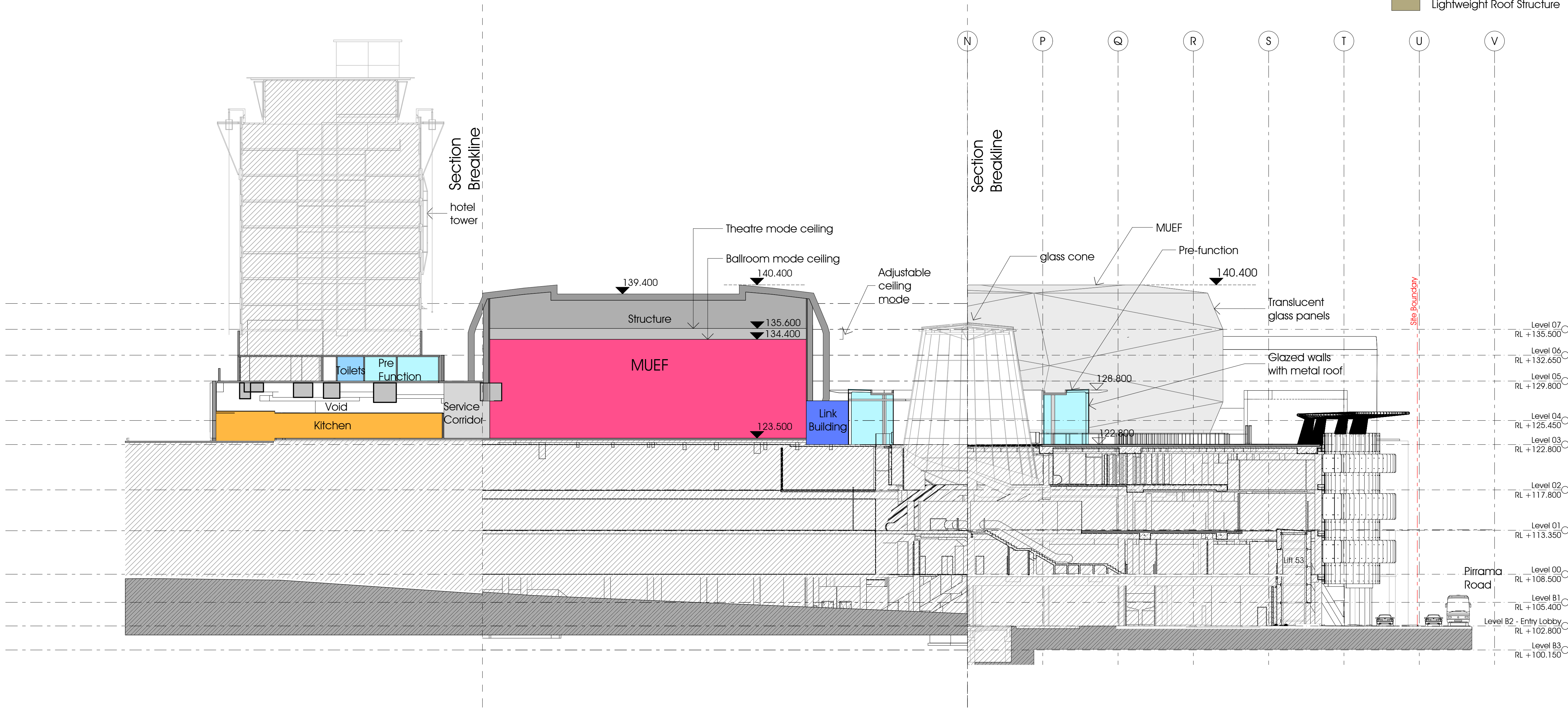
4 Section BB 1:250
