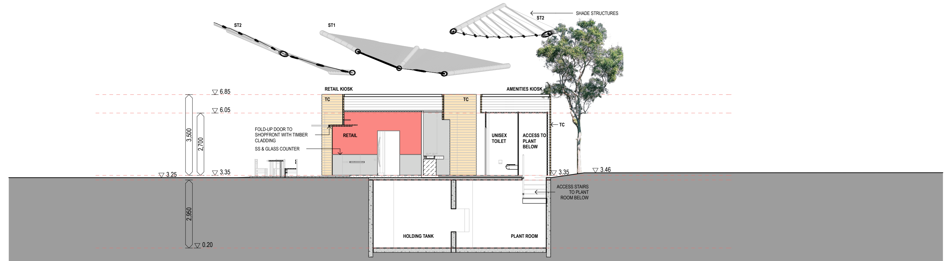
Kiosks Interior 1:100
