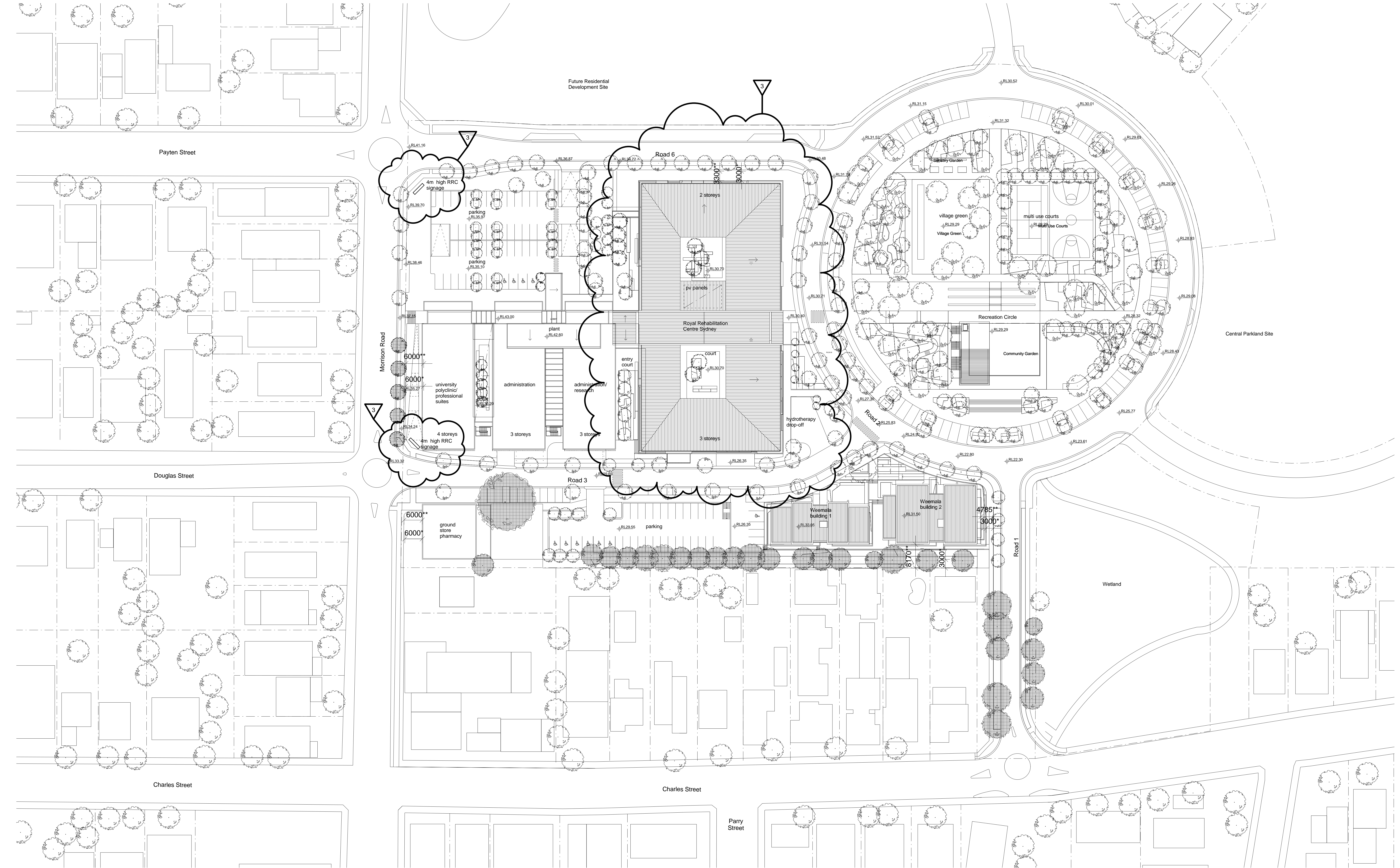
1 SITE PLAN 1:500
