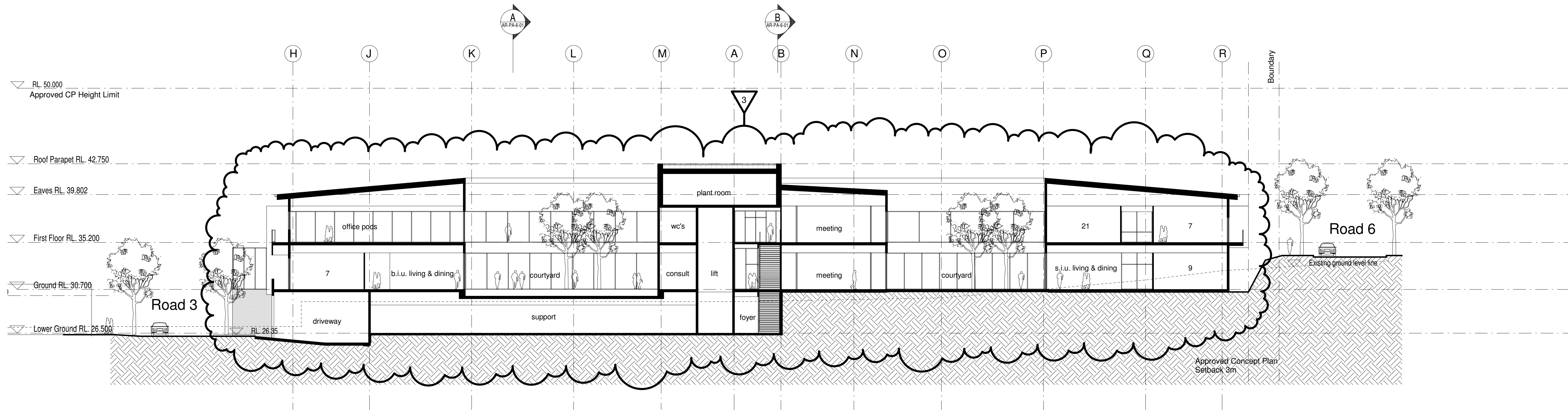
2 SECTION DD 1:200
