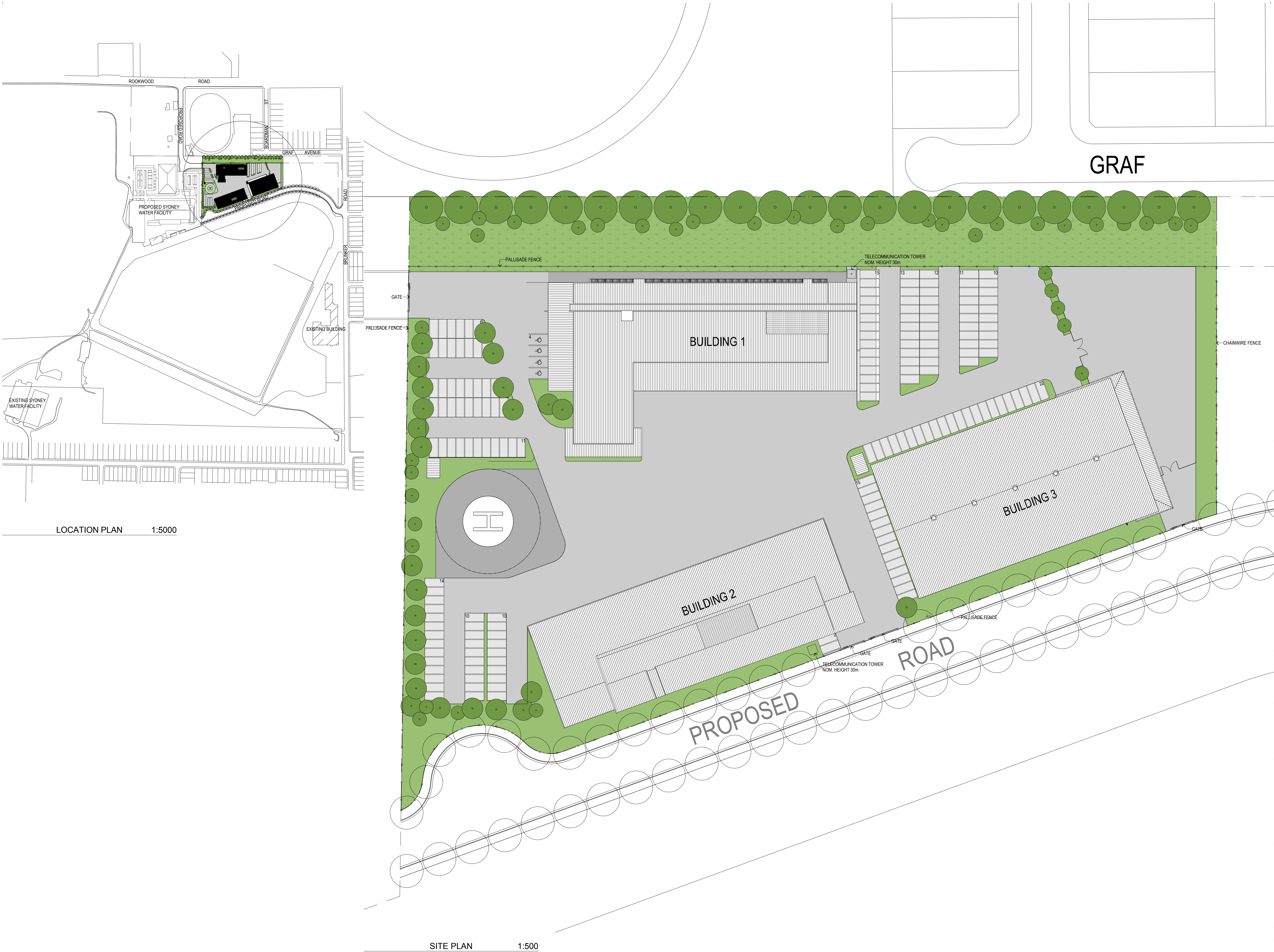
SITE PLAN 1:500
