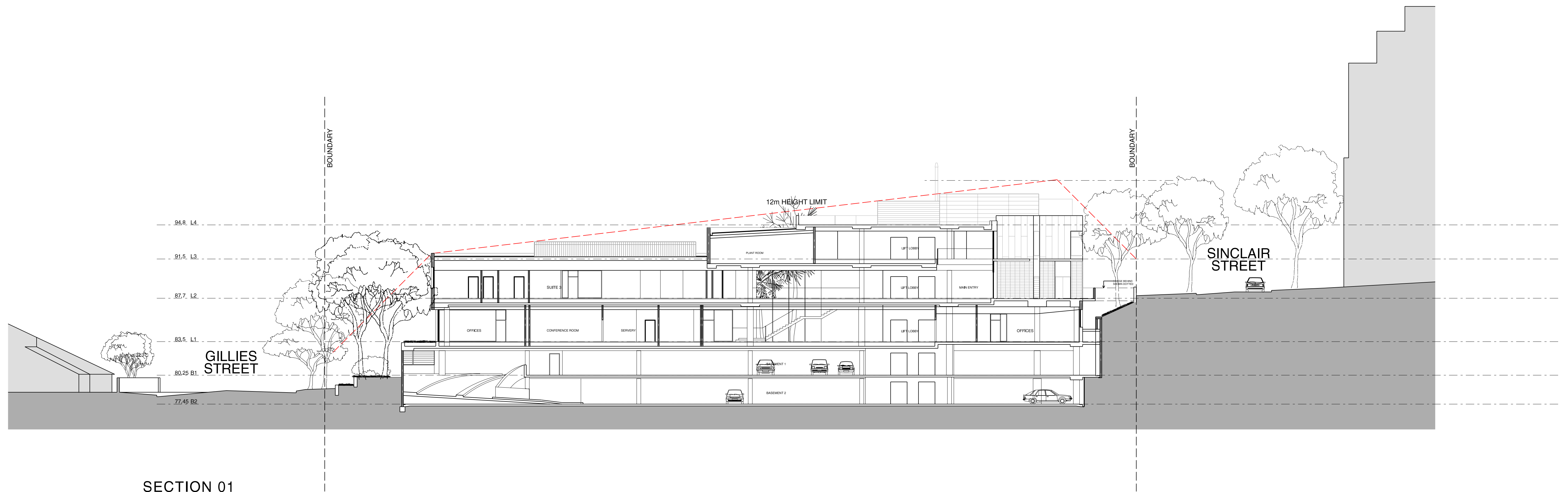
SECTION 01
