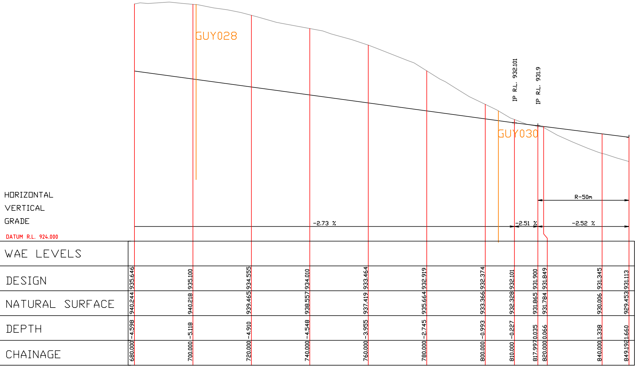
LONGITUDINAL SECTION – ACCESS RD CL
