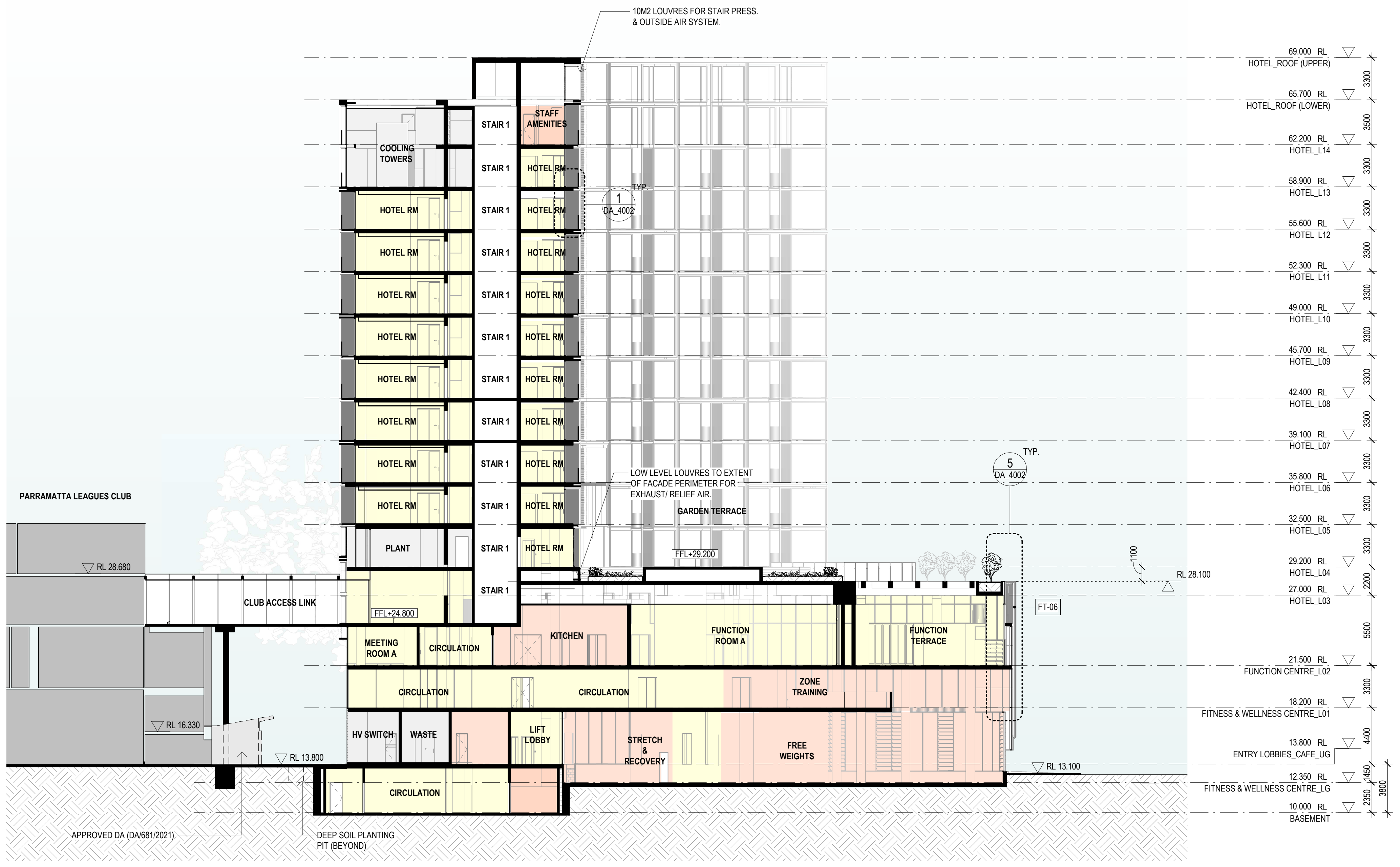
1 GA SECTION 1 DA_1100 1:200
