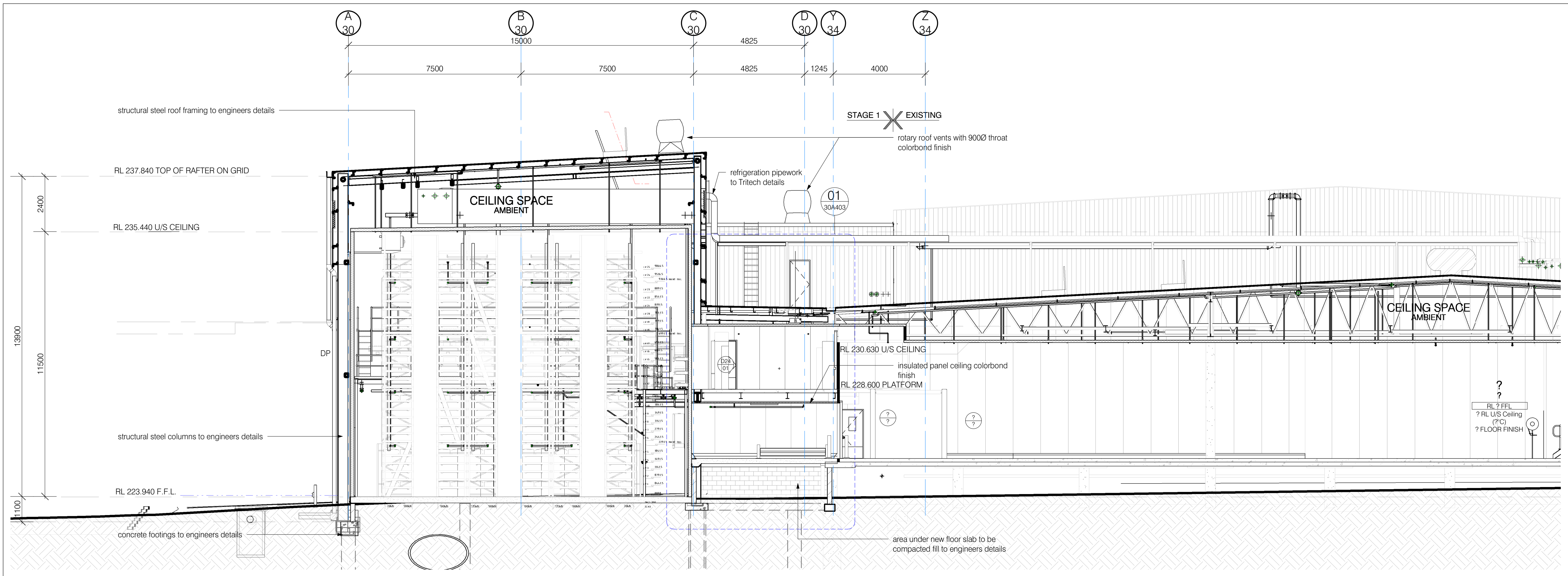
02 SECTION A1 = 1:100
