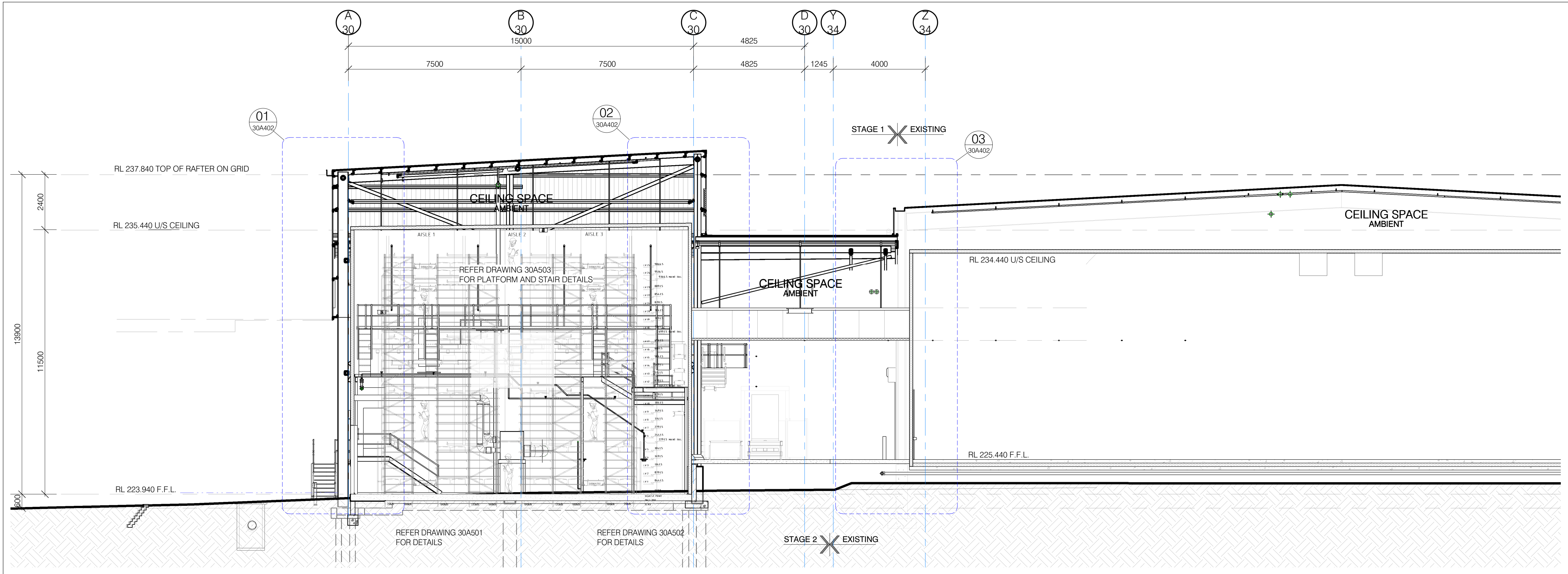
01 SECTION A1 = 1:100
