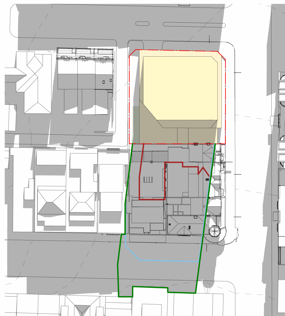
3 ENVELOPE - SHADOWS - 11am 1 : 700
