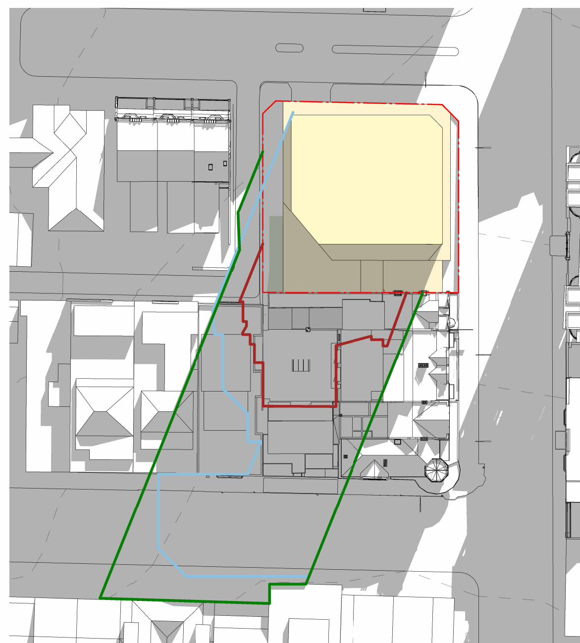
2 ENVELOPE - SHADOWS - 10am 1 : 700
