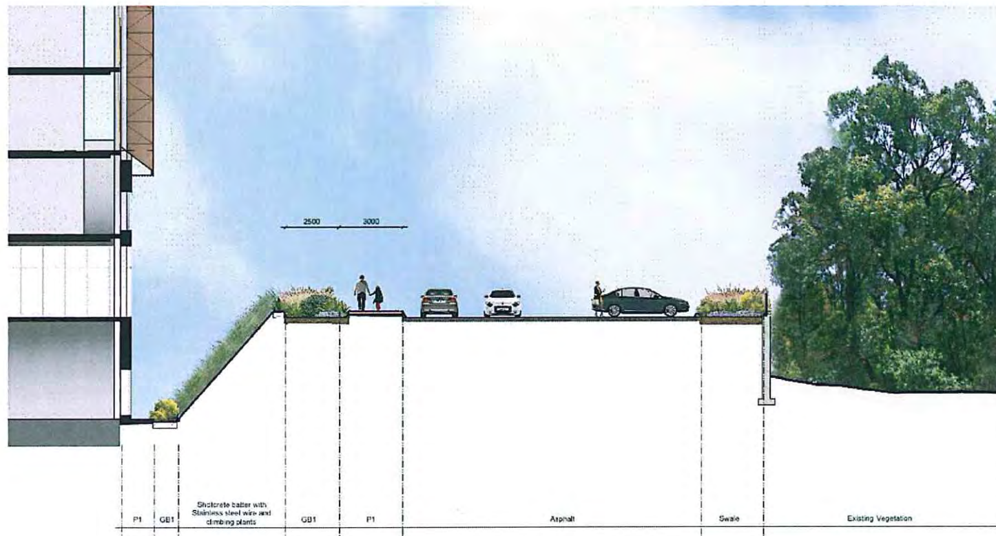
5 Section 5 1:100
