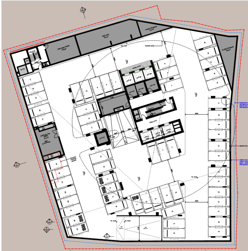
Basement 01
