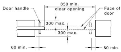
(b) Cavity sliding door
