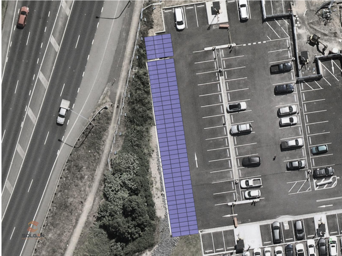
SITE LAYOUT NTS
