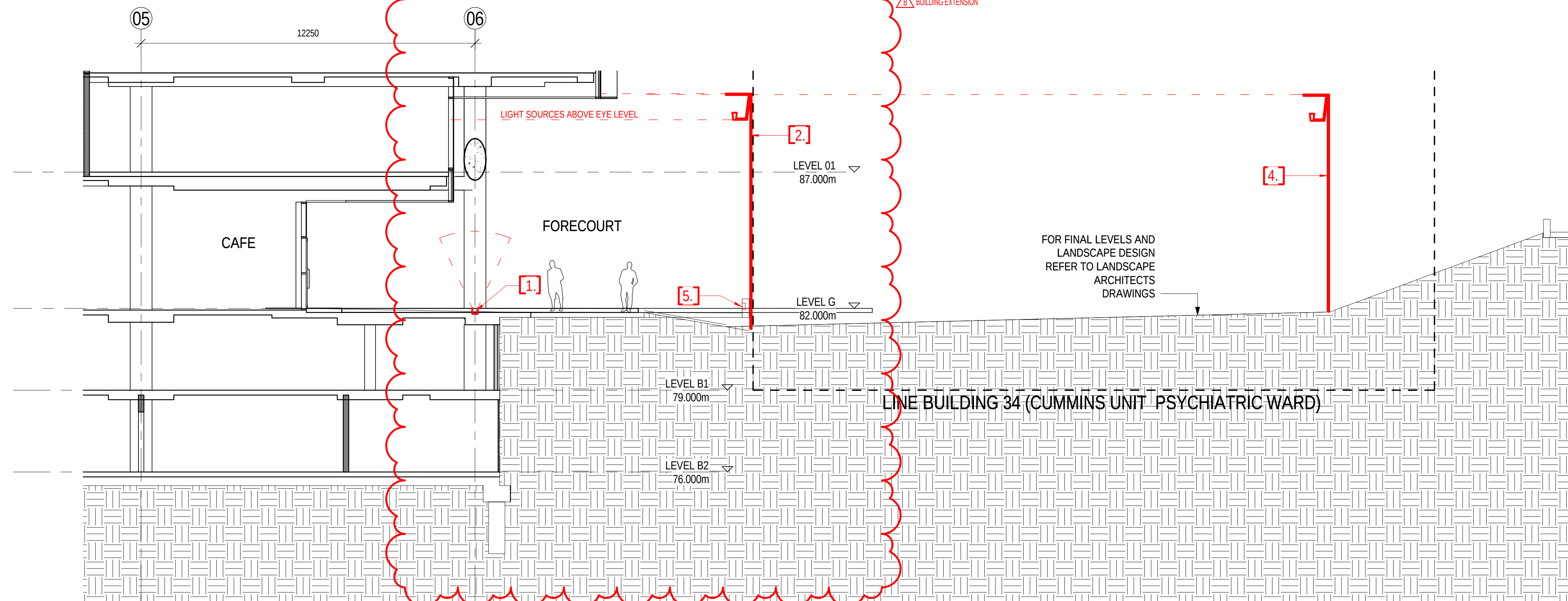
2 SITE SECTION - B
