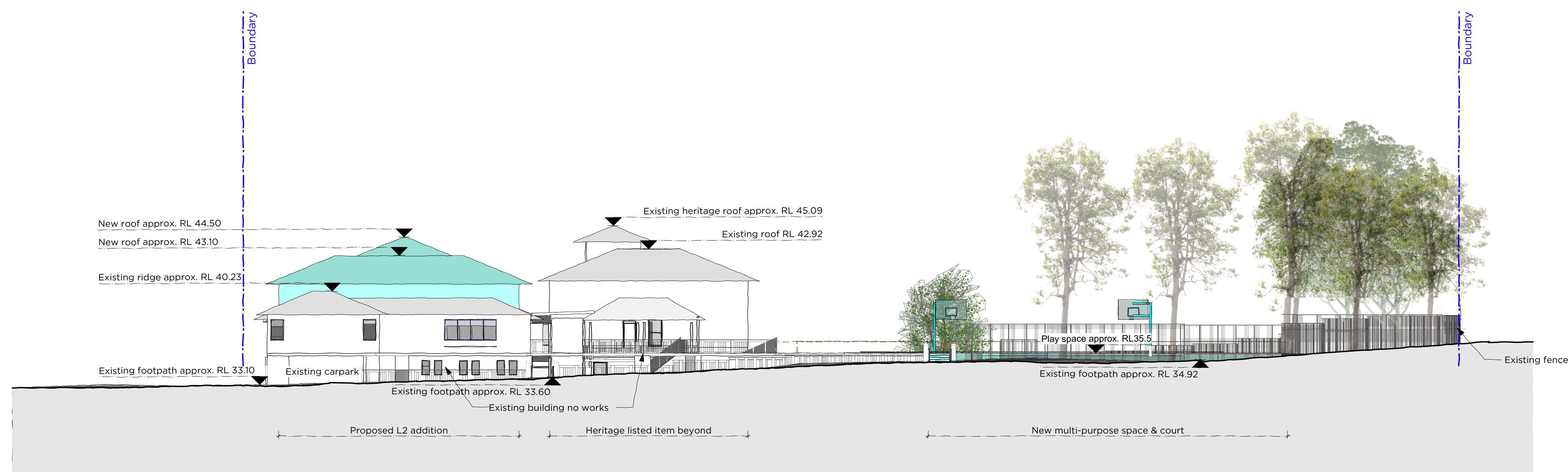
2 Bligh St Elevation Scale: 1:200
