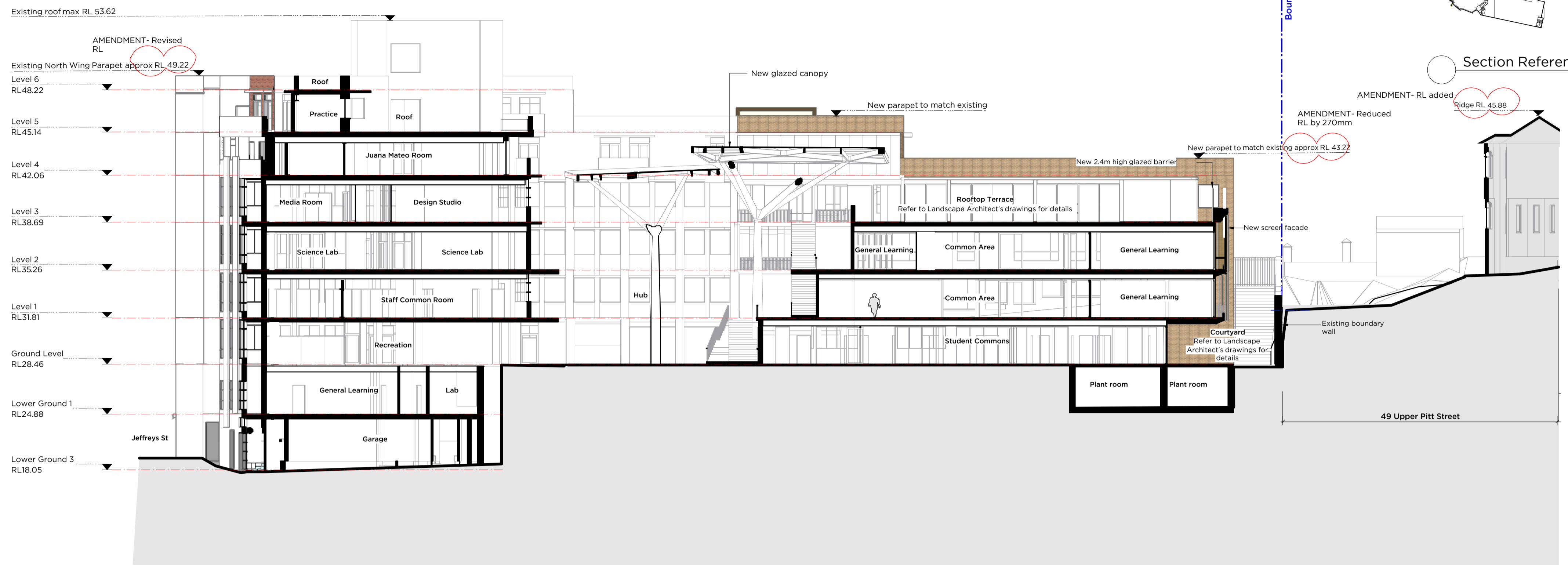
1 Section 1 Scale: 1:200
