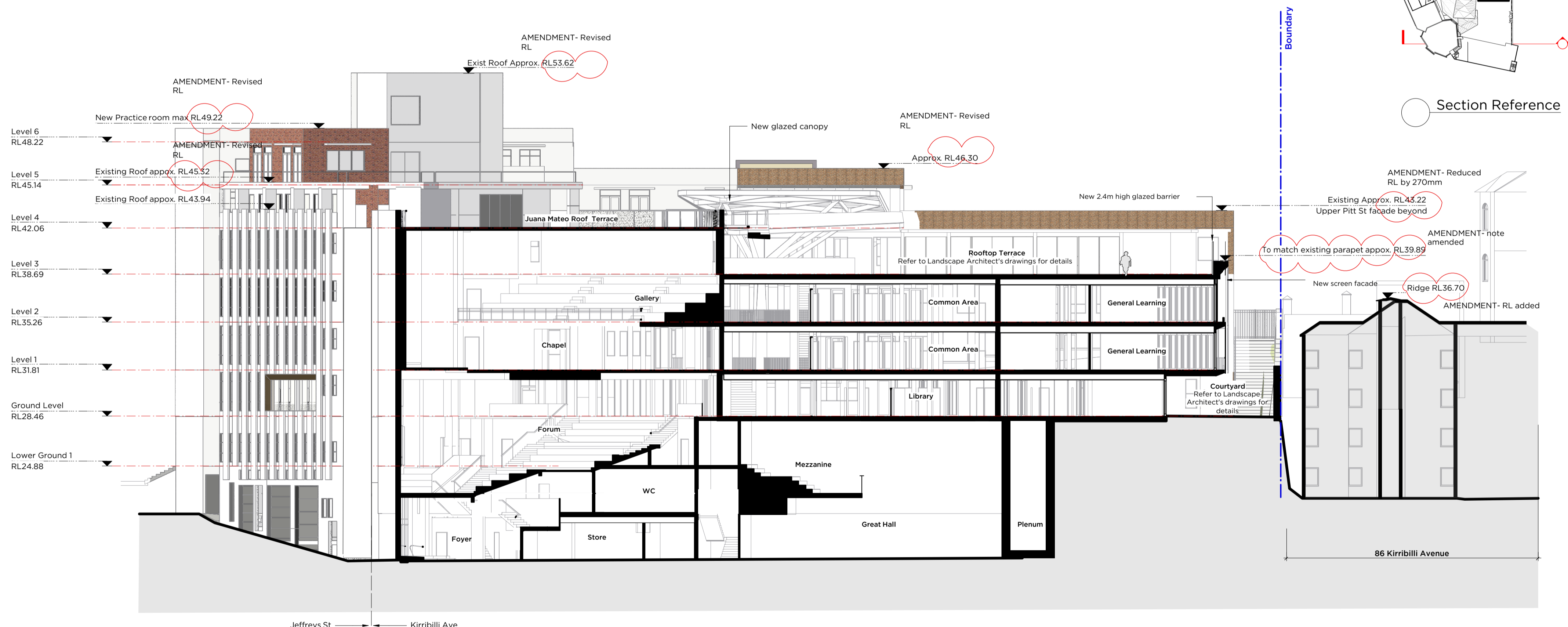
2 Section 2 Scale: 1:200
