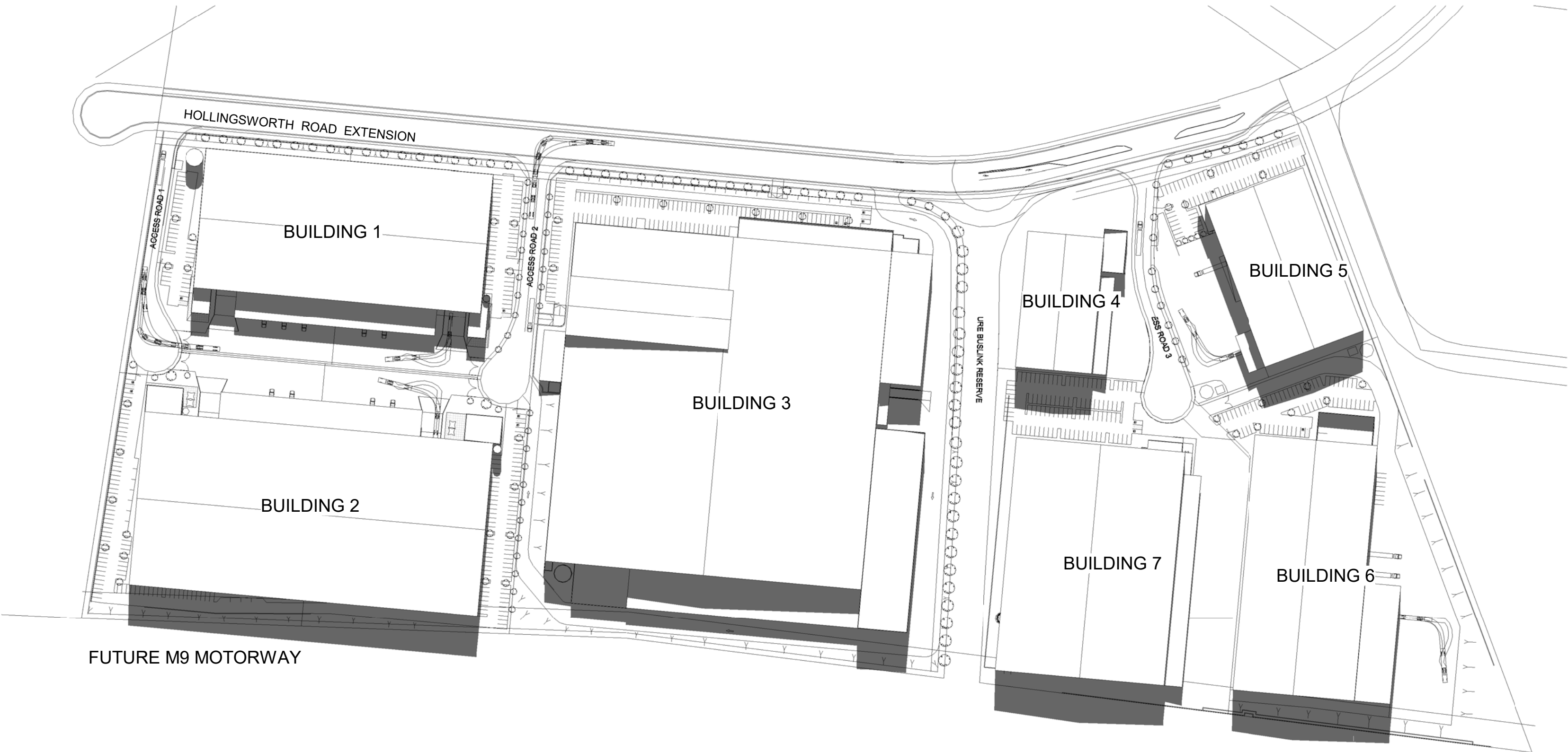
3 21 Jun - 3pm 1 : 2000
