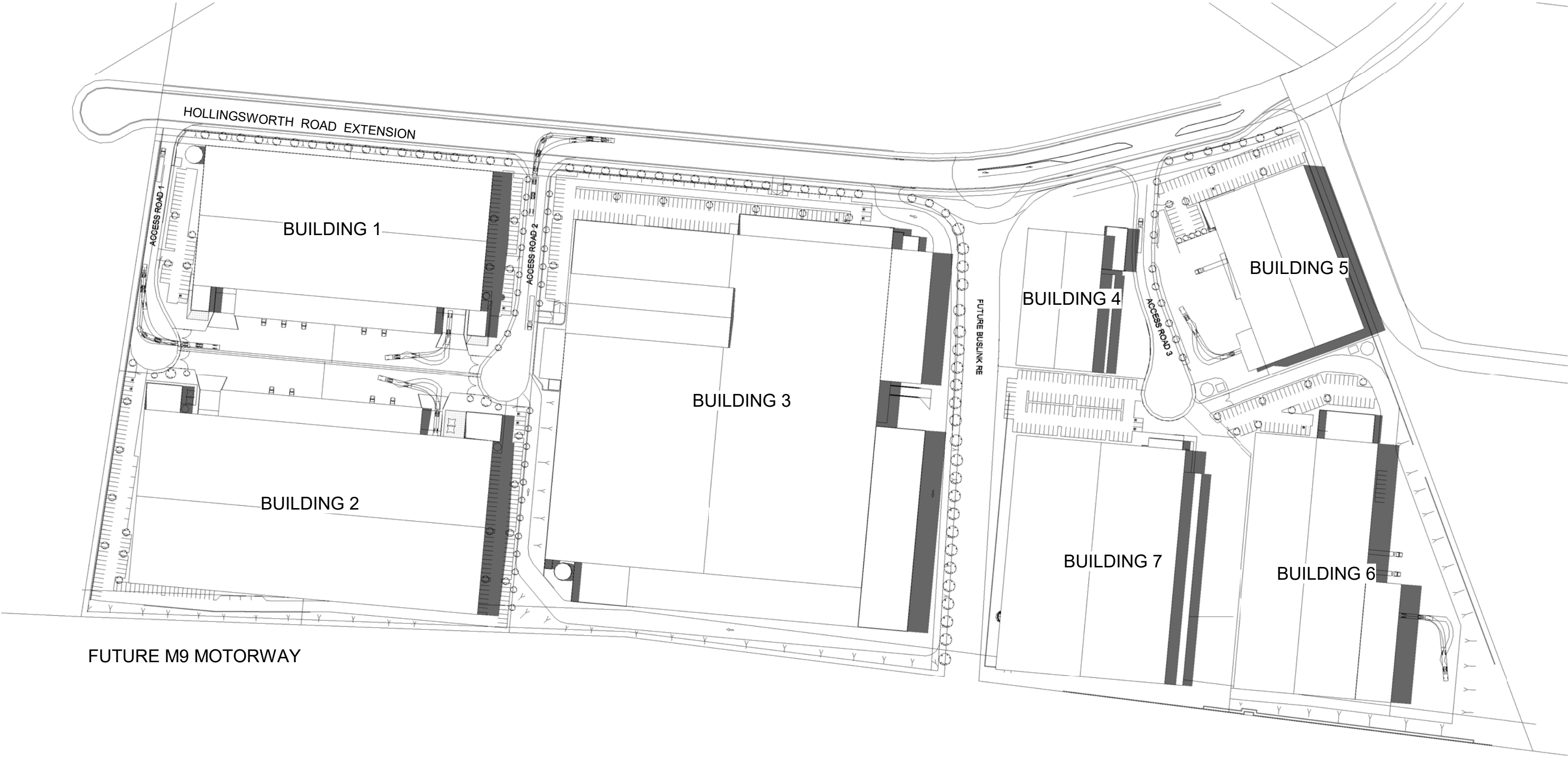
3 21 Dec - 3pm 1 : 2000
